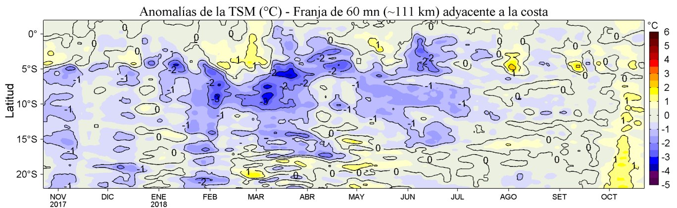
Figura 4. Variación promedio de las anomalías de la temperatura superficial del mar (°C) para una franja de 60 mn (~111 km) adyacente al litoral peruano para los últimos doce meses al 22 de octubre de 2018. Datos: OSTIA-UKMO-L4-GLOB-v2.0 (UK Met Office, 2012; Donlon et al, 2012) disponible en https://podaac.jpl.nasa.gov/dataset/OSTIA-UKMO-L4-GLOB-v2.0 . Las anomalías se calcularon con respecto al periodo 2007-2016. Procesamiento: LHF/AFIOF/DGIOCC/IMARPE.
