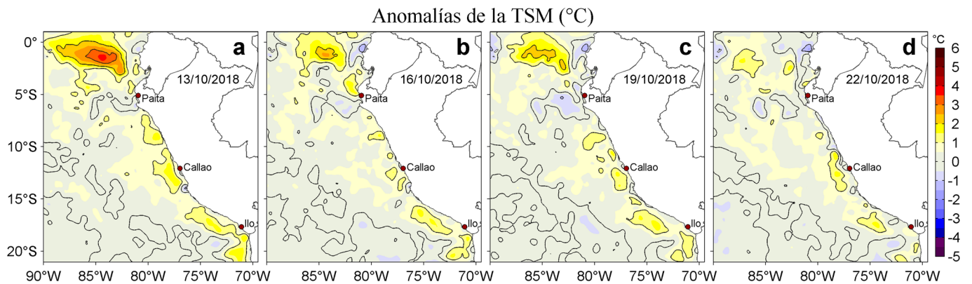
Figura 3. Anomalías de la temperatura superficial del mar (°C) para los días: a) 13, b) 16, c) 19 y d) 22 de octubre de 2018. Las anomalías se calcularon respecto de la climatología para el periodo 2007-2016. Datos: OSTIA-UKMO-L4-GLOB-v2.0 (UK Met Office, 2012; Donlon et al, 2012). Procesamiento: LHF/AFIOF/DGIOCC/IMARPE.
