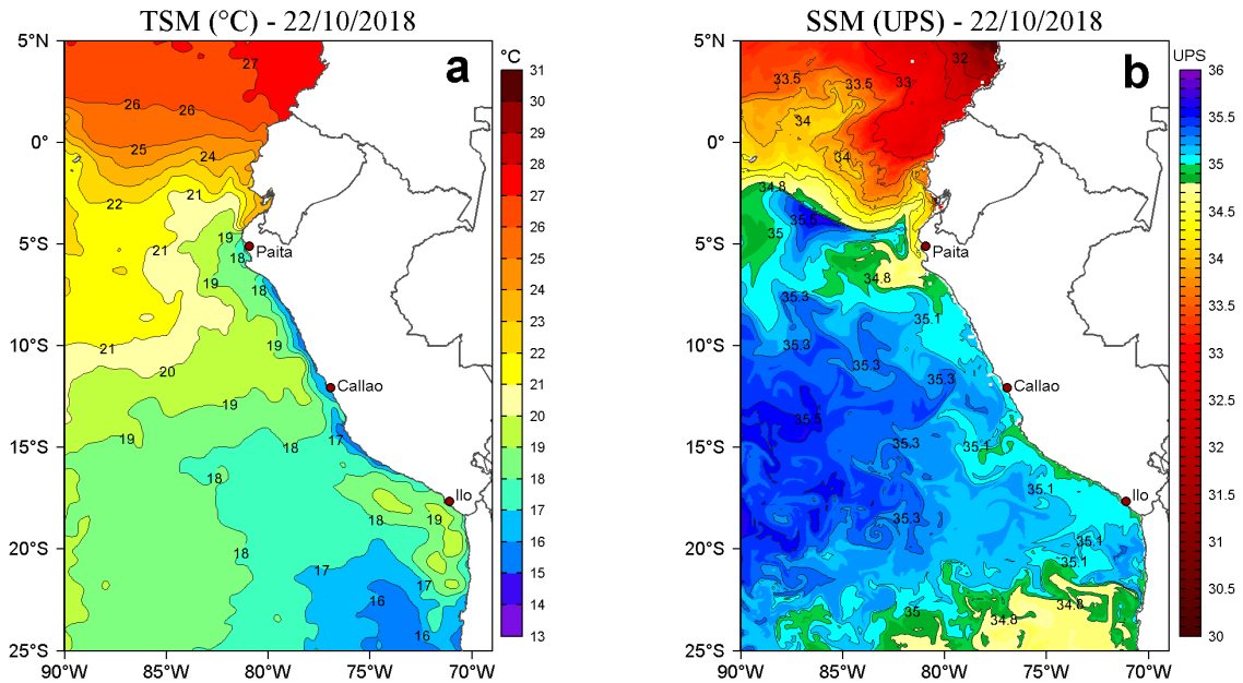
Figura 2. a) Temperatura superficial del mar (°C) y b) Salinidad superficial del mar (UPS) para el 22 de octubre de 2018. Datos: OSTIA-UKMO-L4-GLOB-v2.0 (UK Met Office, 2012; Donlon et al, 2012) disponible en https://podaac.jpl.nasa.gov/dataset/OSTIA-UKMO-L4-GLOB-v2.0 para (a) y Hybrid Coordinate Ocean Model (HYCOM; Halliwell et al., 1998; 2000; Bleck, 2001) para (b). Procesamiento: LHF/AFIOF/DGIOCC/IMARPE.
