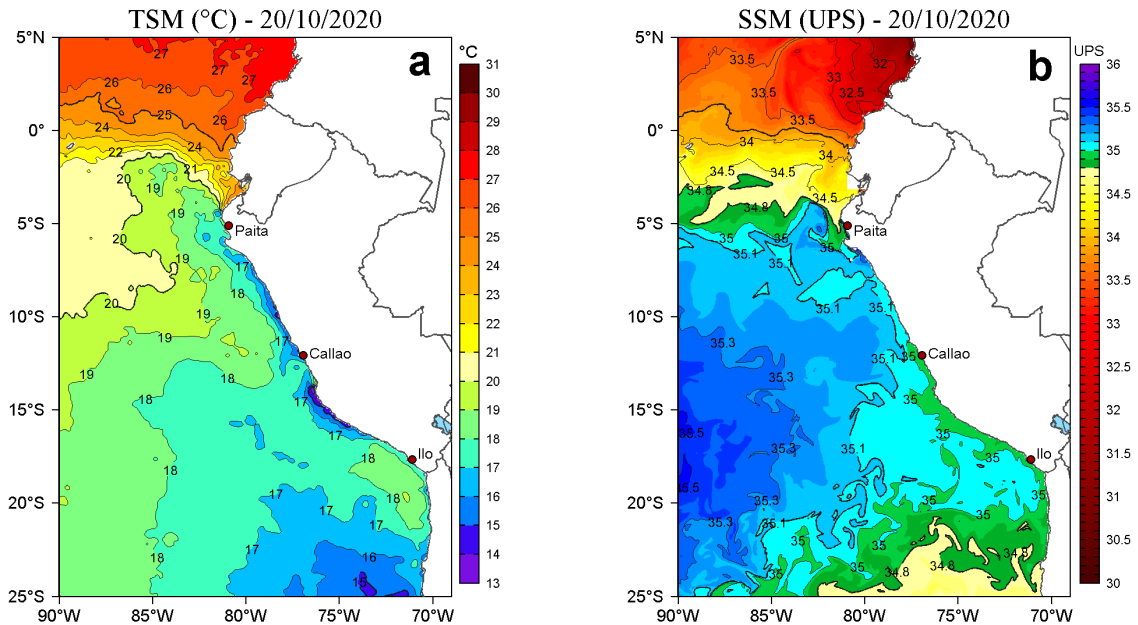
Figura 2. a) Temperatura superficial del mar (TSM, °C) y b) Salinidad superficial del mar (SSM, UPS), para el 20 de octubre de 2020. Datos: OSTIA-UKMO-L4-GLOB-v2.0 (UK Met Office, 2012; Donlon et al, 2012) disponible en https://podaac.jpl.nasa.gov/dataset/OSTIA-UKMO-L4-GLOB-v2.0 para (a) y Hybrid Coordinate Ocean Model v. GOFS 3.1 (HYCOM; Halliwell et al., 1998; 2000; Bleck, 2001) para (b). Procesamiento: LHFM/AFIOF/DGIOCC.
