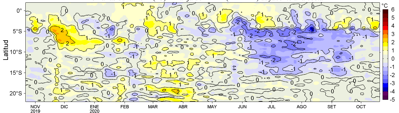
Figura 4. Variación promedio de las anomalías de la temperatura superficial del mar (TSM, °C) para una franja de 60 mn (~111 km) adyacente al litoral peruano para los últimos doce meses al 20 de octubre de 2020. Datos: OSTIA-UKMO-L4-GLOB-v2.0 (UK Met. Office, 2012; Donlon et al, 2012) disponible en https://podaac.jpl.nasa.gov/dataset/OSTIA-UKMO-L4-GLOB-v2.0 . Las anomalías se calcularon con respecto al periodo 2007-2016. Procesamiento: LHFM/AFIOF/DGIOCC.
