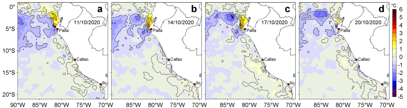
Figura 3. Anomalías de la temperatura superficial del mar (TSM, °C) para los días: a) 11, b) 14, c) 17 y d) 20 de octubre de 2020. Las anomalías se calcularon respecto de la climatología para el periodo 2007-2016. Datos: OSTIA-UKMO-L4-GLOB-v2.0 (UK Met Office, 2012; Donlon et al, 2012). Procesamiento: LHFM/AFIOF/DGIOCC.
