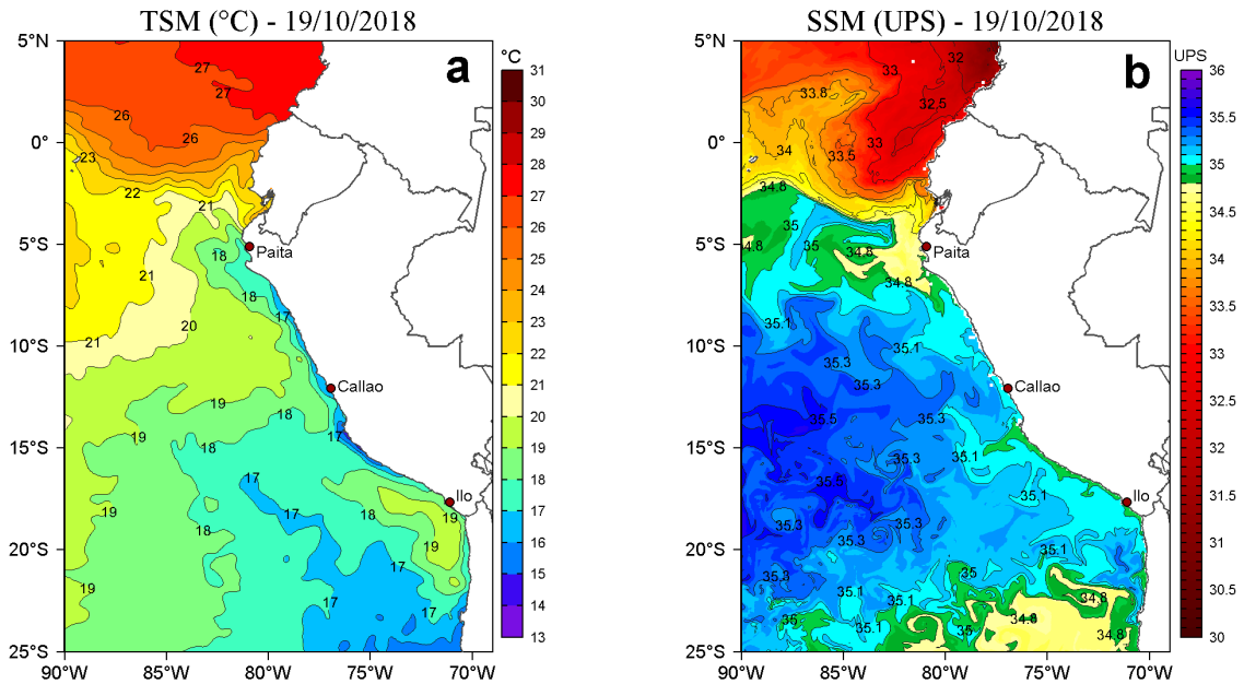
Figura 2. a) Temperatura superficial del mar (°C) y b) Salinidad superficial del mar (UPS) para el 19 de octubre de 2018. Datos: OSTIA-UKMO-L4-GLOB-v2.0 (UK Met Office, 2012; Donlon et al, 2012) disponible en https://podaac.jpl.nasa.gov/dataset/OSTIA-UKMO-L4-GLOB-v2.0 para (a) y Hybrid Coordinate Ocean Model (HYCOM; Halliwell et al., 1998; 2000; Bleck, 2001) para (b). Procesamiento: LHF/AFIOF/DGIOCC/IMARPE.
