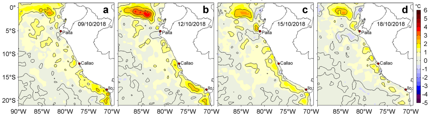
Figura 3. Anomalías de la temperatura superficial del mar ( ^{\circ}\text{C} ) para los días: a) 09, b) 12, c) 15 y d) 18 de octubre de 2018. Las anomalías se calcularon respecto de la climatología para el periodo 2007-2016. Datos: OSTIA-UKMO-L4-GLOB-v2.0 (UK Met Office, 2012; Donlon et al, 2012). Procesamiento: LHF/AFIOF/DGIOCC/IMARPE.
