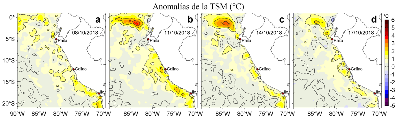
Figura 3. Anomalías de la TSM (°C) para los días: a) 08, b) 11, c) 14 y d) 17 de octubre de 2018. Las anomalías se calcularon respecto de la climatología para el periodo 2007-2016. Datos: OSTIA-UKMO-L4-GLOB-v2.0 (UK Met Office, 2012; Donlon et al, 2012). Procesamiento: LHF/AFIOF/DGIOCC/IMARPE.
