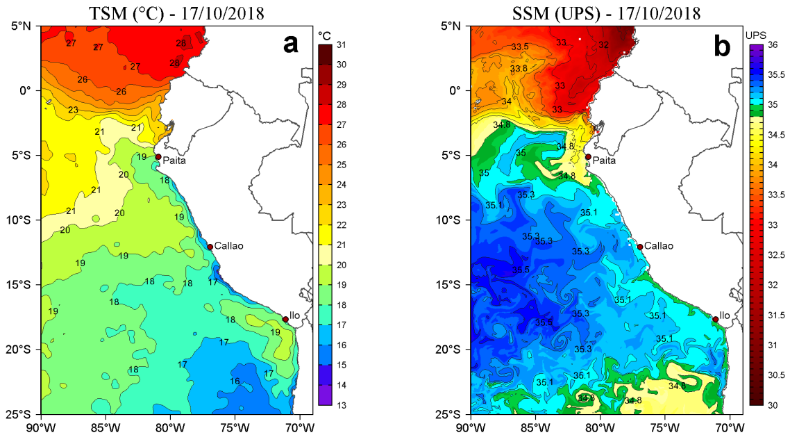
Figura 2. a) Temperatura superficial del mar (TSM, °C) y b) Salinidad superficial del mar (SSM, UPS) para el 17 de octubre de 2018. Datos: OSTIA-UKMO-L4-GLOB-v2.0 (UK Met Office, 2012; Donlon et al, 2012) disponible en https://podaac.jpl.nasa.gov/dataset/OSTIA-UKMO-L4-GLOB-v2.0 ) para (a) y Hybrid Coordinate Ocean Model (HYCOM; Halliwell et al., 1998; 2000; Bleck, 2001) para (b). Procesamiento: LHF/AFIOF/DGIOCC/IMARPE.
