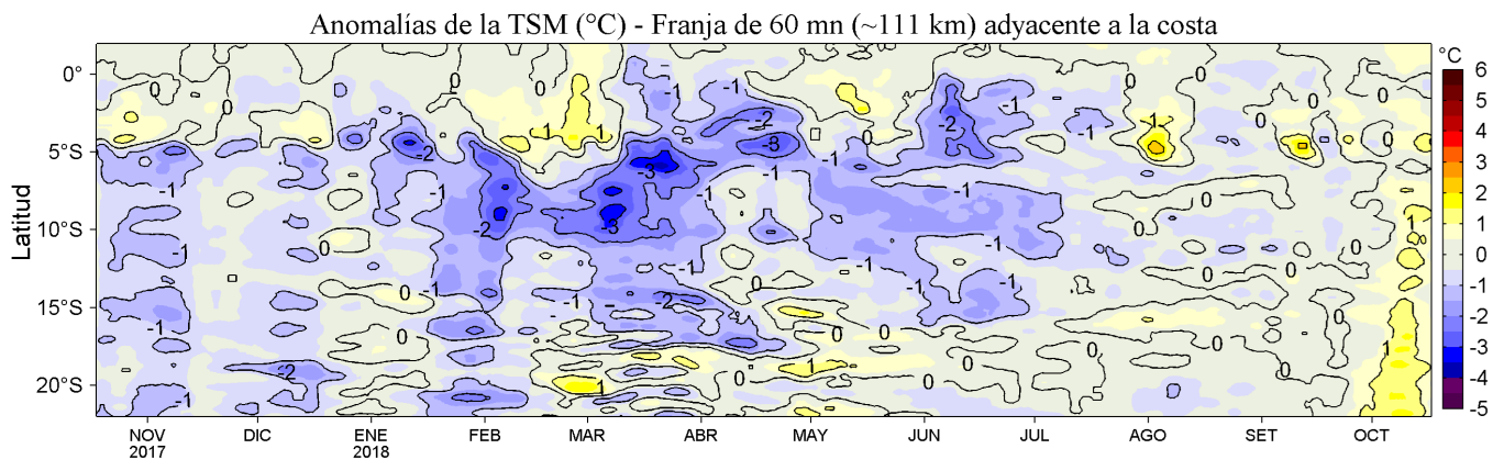
Figura 4. Variación promedio de las anomalías de la TSM (°C) para una franja de 60 mn (~111 km) adyacente al litoral peruano para los últimos doce meses al 17 de octubre de 2018. Datos: OSTIA-UKMO-L4-GLOB-v2.0 (UK Met. Office, 2012; Donlon et al, 2012) disponible en https://podaac.jpl.nasa.gov/dataset/OSTIA-UKMO-L4-GLOB-v2.0 ). Las anomalías se calcularon con respecto al periodo 2007-2016. Procesamiento: LHF/AFIOF/DGIOCC/IMARPE.
