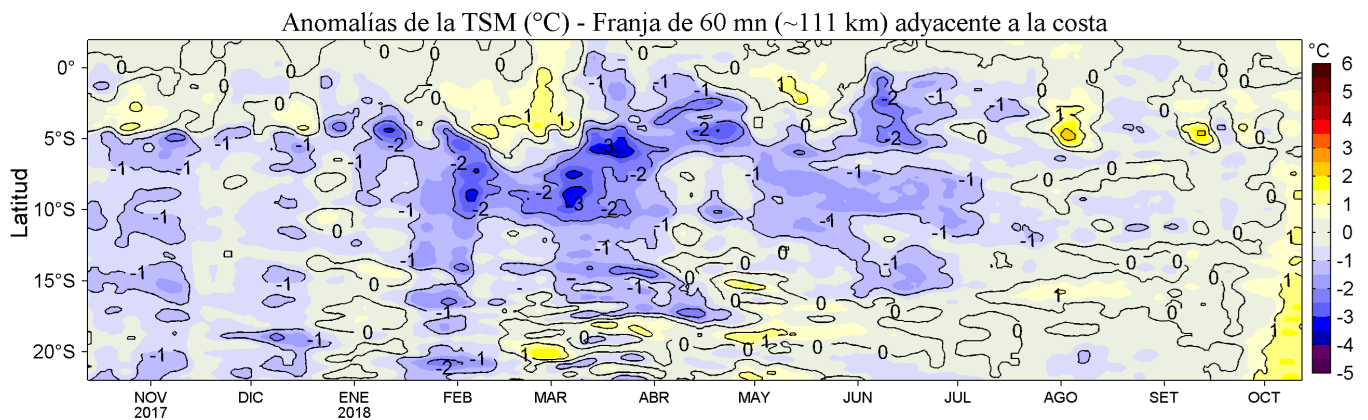
Figura 4. Variación promedio de las anomalías de la temperatura superficial del mar TSM (°C) para una franja de 60 mn (~111 km) adyacente al litoral peruano para los últimos doce meses al 12 de octubre de 2018. Datos: OSTIA-UKMO-L4-GLOB-v2.0 (UK Met. Office, 2012; Donlon et al, 2012) disponible en https://podaac.jpl.nasa.gov/dataset/OSTIA-UKMO-L4-GLOB-v2.0 ). Las anomalías se calcularon con respecto al periodo 2007-2016. Procesamiento: LHF/AFIOF/DGIOCC/IMARPE.
