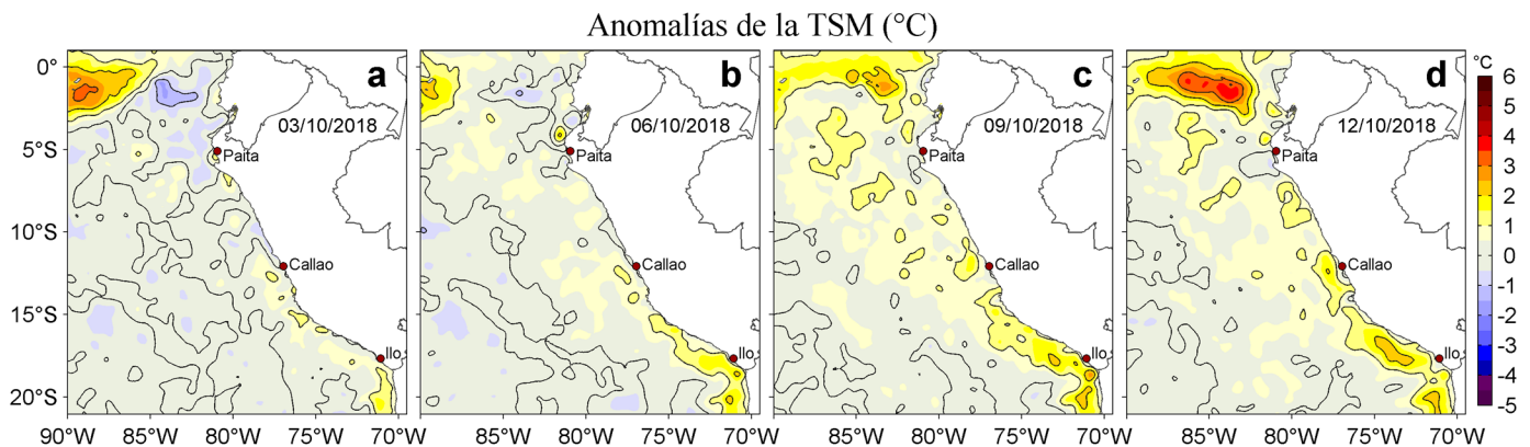
Figura 3. Anomalías de la temperatura superficial del mar TSM (°C) para los días: a) 03, b) 06, c) 09 y d) 12 de octubre de 2018. Las anomalías se calcularon respecto de la climatología para el periodo 2007-2016. Datos: OSTIA-UKMO-L4-GLOB-v2.0 (UK Met Office, 2012; Donlon et al, 2012). Procesamiento: LHF/AFIOF/DGIOCC/IMARPE.
