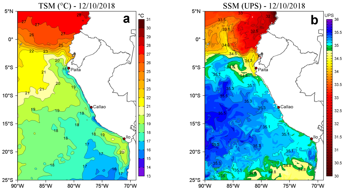
Figura 2. a) Temperatura superficial del mar (TSM, °C) y b) Salinidad superficial del mar (SSM, UPS) para el 12 de octubre de 2018. Datos: OSTIA-UKMO-L4-GLOB-v2.0 (UK Met Office, 2012; Donlon et al, 2012) disponible en https://podaac.jpl.nasa.gov/dataset/OSTIA-UKMO-L4-GLOB-v2.0 ) para (a) y Hybrid Coordinate Ocean Model (HYCOM; Halliwell et al., 1998; 2000; Bleck, 2001) para (b). Procesamiento: LHF/AFIOF/DGIOCC/IMARPE.
