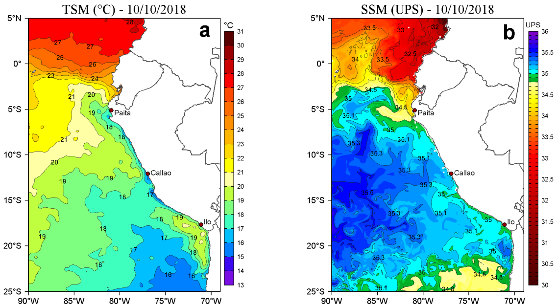
Figura 2. a) Temperatura superficial del mar TSM ( ^{\circ}\text{C} ) y b) Salinidad superficial del mar SSM (UPS) para el 10 de octubre de 2018. Datos: OSTIA-UKMO-L4-GLOB-v2.0 (UK Met Office, 2012; Donlon et al, 2012) disponible en https://podaac.jpl.nasa.gov/dataset/OSTIA-UKMO-L4-GLOB-v2.0 ) para (a) y Hybrid Coordinate Ocean Model (HYCOM; Halliwell et al., 1998; 2000; Bleck, 2001) para (b). Procesamiento: LHF/AFIOF/DGIOCC/IMARPE.
