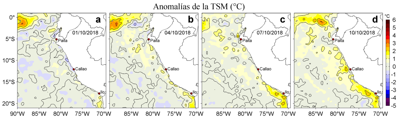
Figura 3. Anomalías de la temperatura superficial del mar TSM ( ^{\circ}\text{C} ) para los días: a) 01, b) 04, c) 07 y d) 10 de octubre de 2018. Las anomalías se calcularon respecto de la climatología para el periodo 2007-2016. Datos: OSTIA-UKMO-L4-GLOB-v2.0 (UK Met Office, 2012; Donlon et al, 2012). Procesamiento: LHF/AFIOF/DGIOCC/IMARPE.
