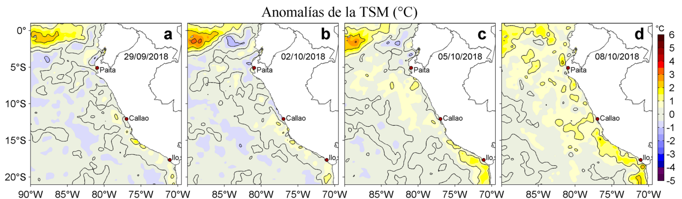
Figura 3. Anomalías de la temperatura superficial del mar TSM ( ^{\circ}\text{C} ) para los días: a) 29 de setiembre y b) 02, c) 05 y d) 08 de octubre de 2018. Las anomalías se calcularon respecto de la climatología para el periodo 2007-2016. Datos: OSTIA-UKMO-L4-GLOB-v2.0 (UK Met Office, 2012; Donlon et al, 2012). Procesamiento: LHF/AFIOF/DGIOCC/IMARPE.
