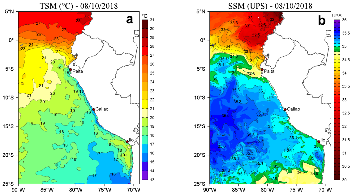
Figura 2. a) Temperatura superficial del mar TSM ( ^{\circ}\text{C} ) y b) Salinidad superficial del mar SSM (UPS) para el 08 de octubre de 2018. Datos: OSTIA-UKMO-L4-GLOB-v2.0 (UK Met Office, 2012; Donlon et al, 2012) disponible en https://podaac.jpl.nasa.gov/dataset/OSTIA-UKMO-L4-GLOB-v2.0 ) para (a) y Hybrid Coordinate Ocean Model (HYCOM; Halliwell et al., 1998; 2000; Bleck, 2001) para (b). Procesamiento: LHF/AFIOF/DGIOCC/IMARPE.
