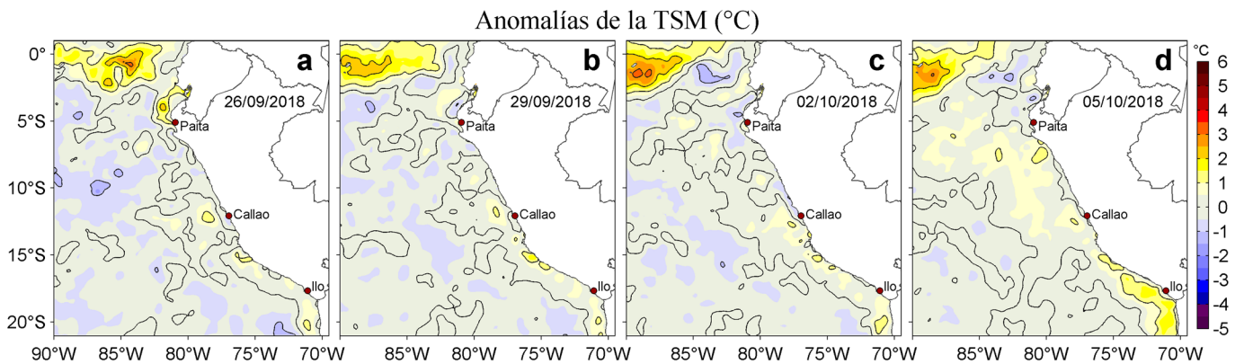
Figura 3. Anomalías de la temperatura superficial del mar TSM ( ^{\circ}\text{C} ) para los días: a) 26 y b) 29 de setiembre, c) 02 y d) 05 de octubre de 2018. Las anomalías se calcularon respecto de la climatología para el periodo 2007-2016. Datos: OSTIA-UKMO-L4-GLOB-v2.0 (UK Met Office, 2012; Donlon et al, 2012). Procesamiento: LHF/AFIOF/DGIOCC/IMARPE.
