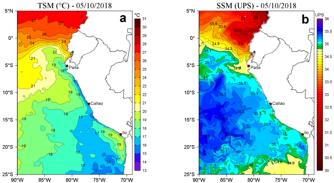
Figura 2. a) Temperatura superficial del mar TSM ( ^{\circ}\text{C} ) y b) Salinidad superficial del mar SSM (UPS) para el 05 de octubre de 2018. Datos: OSTIA-UKMO-L4-GLOB-v2.0 (UK Met Office, 2012; Donlon et al, 2012) disponible en https://podaac.jpl.nasa.gov/dataset/OSTIA-UKMO-L4-GLOB-v2.0 ) para (a) y Hybrid Coordinate Ocean Model (HYCOM; Halliwell et al., 1998; 2000; Bleck, 2001) para (b). Procesamiento: LHF/AFIOF/DGIOCC/IMARPE.
