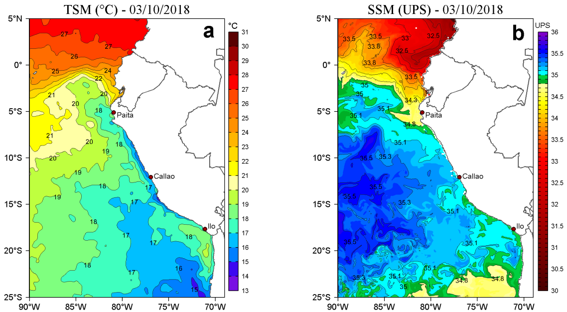
Figura 2. a) Temperatura superficial del mar TSM ( ^{\circ}\text{C} ) y b) Salinidad superficial del mar SSM (UPS) para el 03 de octubre de 2018. Datos: OSTIA-UKMO-L4-GLOB-v2.0 (UK Met Office, 2012; Donlon et al, 2012) disponible en https://podaac.jpl.nasa.gov/dataset/OSTIA-UKMO-L4-GLOB-v2.0 ) para (a) y Hybrid Coordinate Ocean Model (HYCOM; Halliwell et al., 1998; 2000; Bleck, 2001) para (b). Procesamiento: LHF/AFIOF/DGIOCC/IMARPE.
