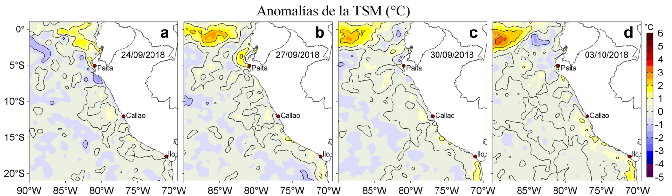
Figura 3. Anomalías de la temperatura superficial del mar TSM ( ^{\circ}\text{C} ) para los días: a) 24, b) 27 y c) 30 de setiembre y d) 03 de octubre de 2018. Las anomalías se calcularon respecto de la climatología para el periodo 2007-2016. Datos: OSTIA-UKMO-L4-GLOB-v2.0 (UK Met Office, 2012; Donlon et al, 2012). Procesamiento: LHF/AFIOF/DGIOCC/IMARPE.
