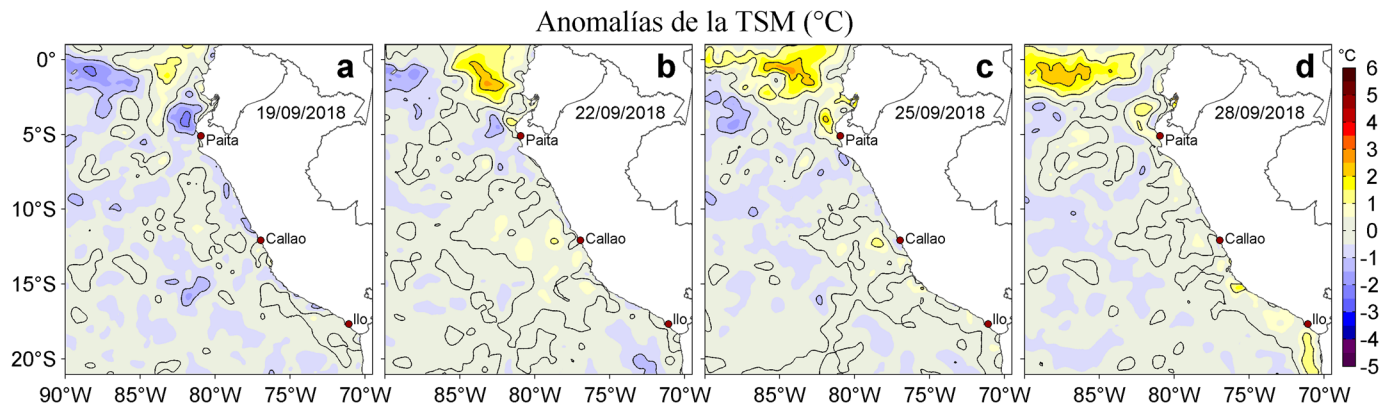
Figura 3. Anomalías de la temperatura superficial del mar TSM ( ^{\circ}\text{C} ) para los días: a) 19, b) 22, c) 25 y d) 28 de setiembre de 2018. Las anomalías se calcularon respecto de la climatología para el periodo 2007-2016. Datos: OSTIA-UKMO-L4-GLOB-v2.0 (UK Met Office, 2012; Donlon et al, 2012). Procesamiento: LHF/AFIOF/DGIOCC/IMARPE.
