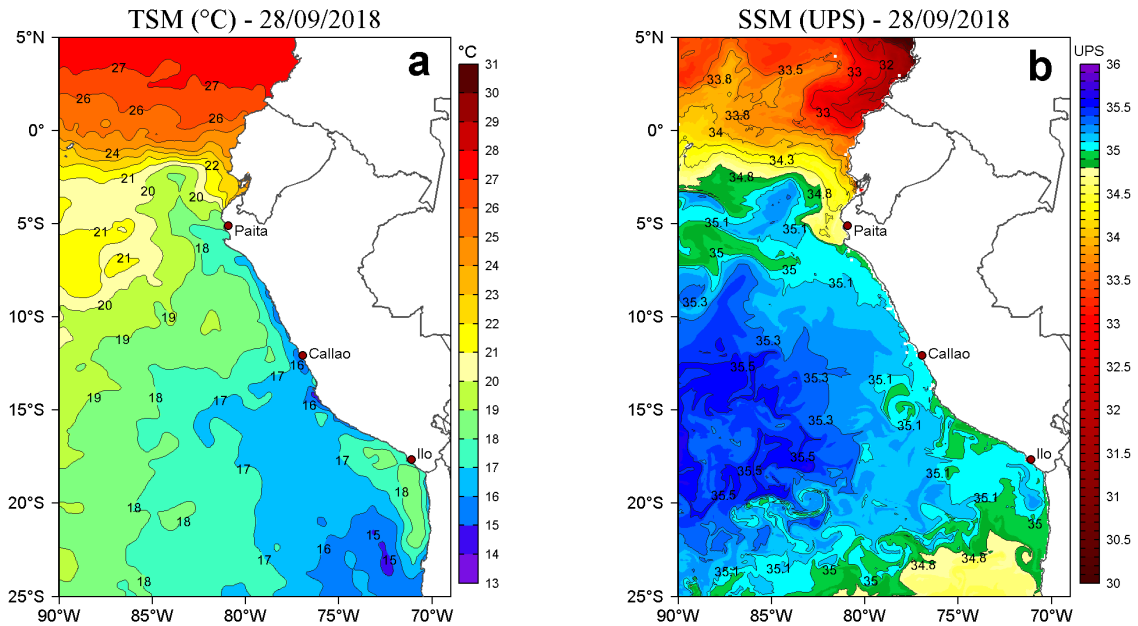
Figura 2. a) Temperatura superficial del mar TSM ( ^{\circ}\text{C} ) y b) Salinidad superficial del mar SSM (UPS) para el 28 de setiembre de 2018. Datos: OSTIA-UKMO-L4-GLOB-v2.0 (UK Met Office, 2012; Donlon et al, 2012) disponible en https://podaac.jpl.nasa.gov/dataset/OSTIA-UKMO-L4-GLOB-v2.0 ) para (a) y Hybrid Coordinate Ocean Model (HYCOM; Halliwell et al., 1998; 2000; Bleck, 2001) para (b). Procesamiento: LHF/AFIOF/DGIOCC/IMARPE.
