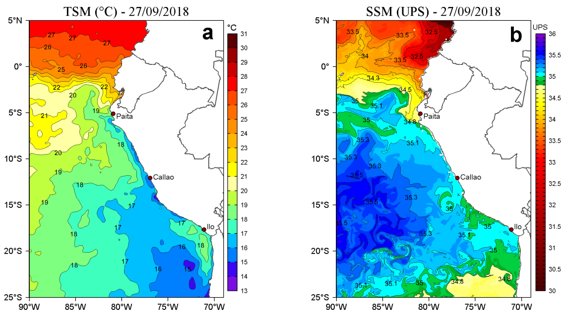
Figura 2. a) Temperatura superficial del mar ( ^{\circ}\text{C} ) y b) Salinidad superficial del mar (UPS) para el 27 de setiembre de 2018. Datos: OSTIA-UKMO-L4-GLOB-v2.0 (UK Met Office, 2012; Donlon et al, 2012) disponible en https://podaac.jpl.nasa.gov/dataset/OSTIA-UKMO-L4-GLOB-v2.0 para (a) y Hybrid Coordinate Ocean Model (HYCOM; Halliwell et al., 1998; 2000; Bleck, 2001) para (b). Procesamiento: LHF/AFIOF/DGIOCC/IMARPE.
