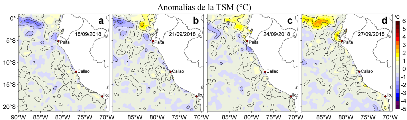
Figura 3. Anomalías de la temperatura superficial del mar ( ^{\circ}\text{C} ) para los días: a) 18, b) 21, c) 24 y d) 27 de setiembre de 2018. Las anomalías se calcularon respecto de la climatología para el periodo 2007-2016. Datos: OSTIA-UKMO-L4-GLOB-v2.0 (UK Met Office, 2012; Donlon et al, 2012). Procesamiento: LHF/AFIOF/DGIOCC/IMARPE.
