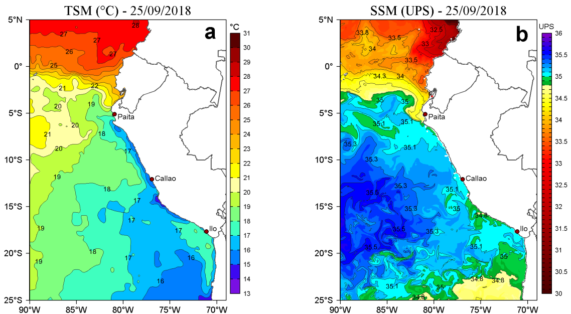
Figura 2. a) Temperatura superficial del mar TSM ( ^{\circ}\text{C} ) y b) Salinidad superficial del mar SSM (UPS) para el 25 de setiembre de 2018. Datos: OSTIA-UKMO-L4-GLOB-v2.0 (UK Met Office, 2012; Donlon et al, 2012) disponible en https://podaac.jpl.nasa.gov/dataset/OSTIA-UKMO-L4-GLOB-v2.0 ) para (a) y Hybrid Coordinate Ocean Model (HYCOM; Halliwell et al., 1998; 2000; Bleck, 2001) para (b). Procesamiento: LHF/AFIOF/DGIOCC/IMARPE.
