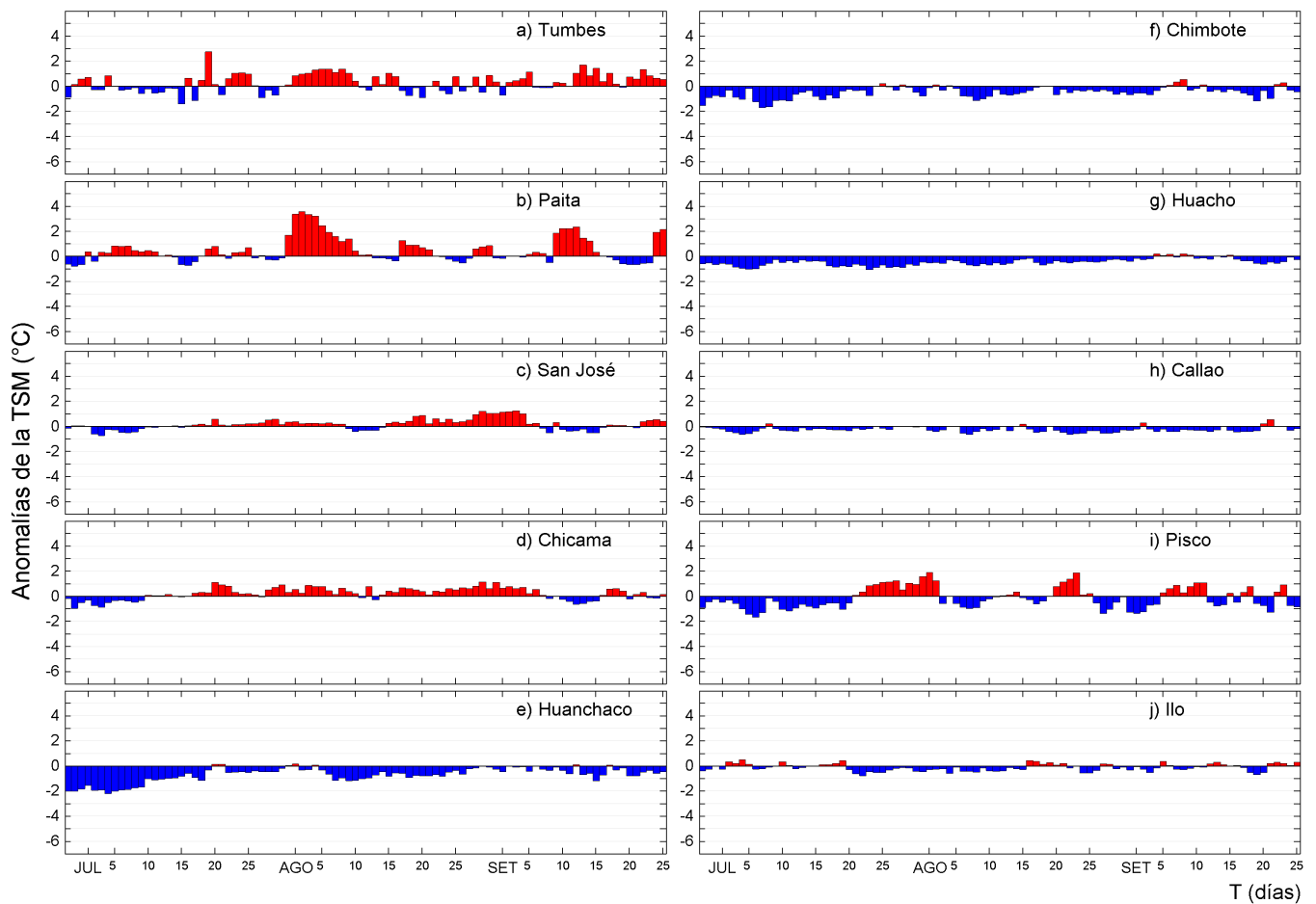
Figura 5. Variación del promedio diario de las anomalías de la temperatura superficial del mar TSM (°C) en la red de estaciones costeras que administra IMARPE en el litoral peruano durante el último trimestre. Las anomalías se calcularon respecto del promedio climatológico pentadal (5 días) para el periodo que se indica en la Tabla 1. Datos y procesamiento: LHFM/AFIOF/DGIOCC/IMARPE.
