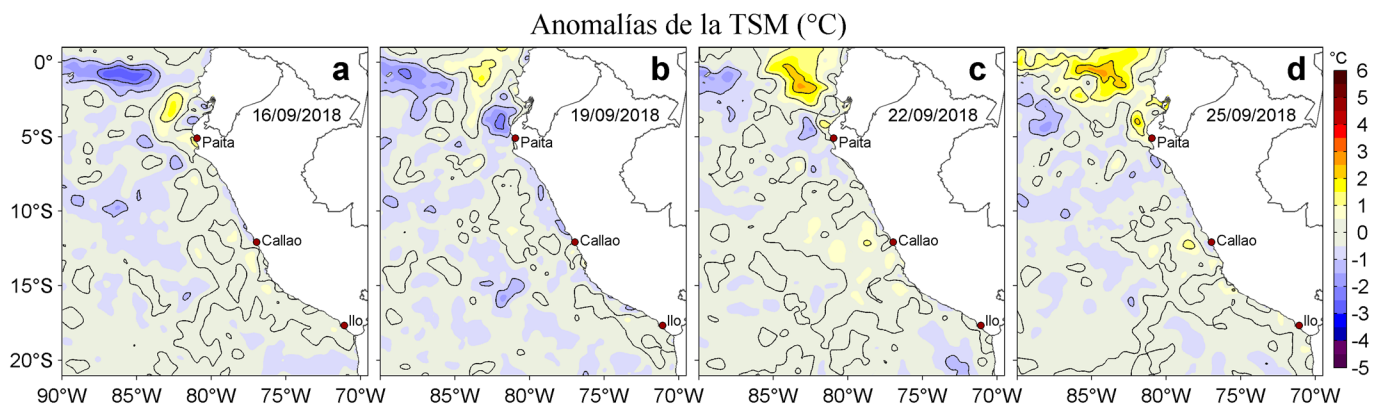
Figura 3. Anomalías de la temperatura superficial del mar TSM ( ^{\circ}\text{C} ) para los días: a) 16, b) 19, c) 22 y d) 25 de setiembre de 2018. Las anomalías se calcularon respecto de la climatología para el periodo 2007-2016. Datos: OSTIA-UKMO-L4-GLOB-v2.0 (UK Met Office, 2012; Donlon et al, 2012). Procesamiento: LHF/AFIOF/DGIOCC/IMARPE.
