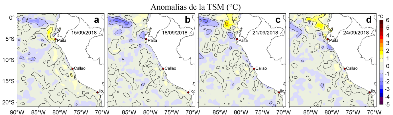
Figura 3. Anomalías de la temperatura superficial del mar TSM ( ^{\circ}\text{C} ) para los días: a) 15, b) 18, c) 21 y d) 24 de setiembre de 2018. Las anomalías se calcularon respecto de la climatología para el periodo 2007-2016. Datos: OSTIA-UKMO-L4-GLOB-v2.0 (UK Met Office, 2012; Donlon et al, 2012). Procesamiento: LHF/AFIOF/DGIOCC/IMARPE.
