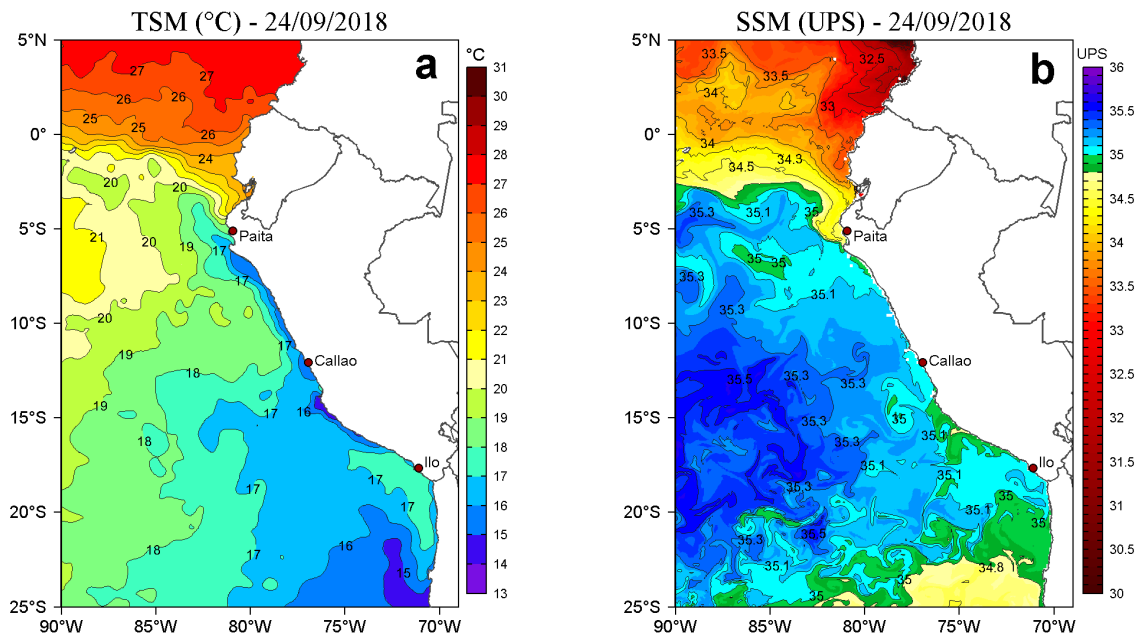
Figura 2. a) Temperatura superficial del mar TSM ( ^{\circ}\text{C} ) y b) Salinidad superficial del mar SSM (UPS) para el 24 de setiembre de 2018. Datos: OSTIA-UKMO-L4-GLOB-v2.0 (UK Met Office, 2012; Donlon et al, 2012) disponible en https://podaac.jpl.nasa.gov/dataset/OSTIA-UKMO-L4-GLOB-v2.0 ) para (a) y Hybrid Coordinate Ocean Model (HYCOM; Halliwell et al., 1998; 2000; Bleck, 2001) para (b). Procesamiento: LHF/AFIOF/DGIOCC/IMARPE.
