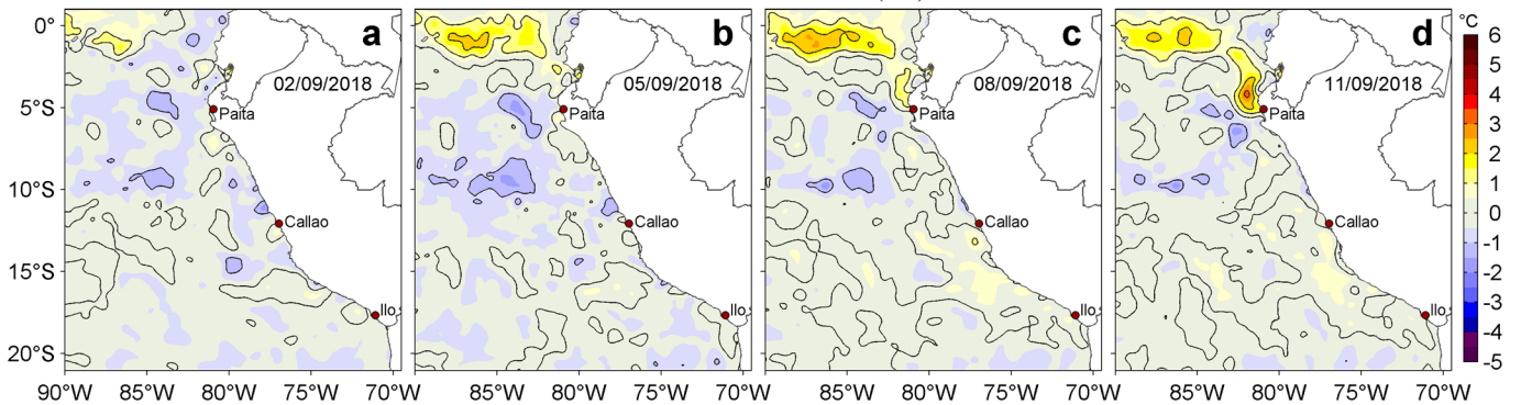
Figura 3. Anomalías de la temperatura superficial del mar TSM ( ^{\circ}\text{C} ) para los días: a) 02, b) 05, c) 08 y d) 11 de setiembre de 2018. Las anomalías se calcularon respecto de la climatología para el periodo 2007-2016. Datos: OSTIA-UKMO-L4-GLOB-v2.0 (UK Met Office, 2012; Donlon et al, 2012). Procesamiento: LHF/AFIOF/DGIOCC/IMARPE.
