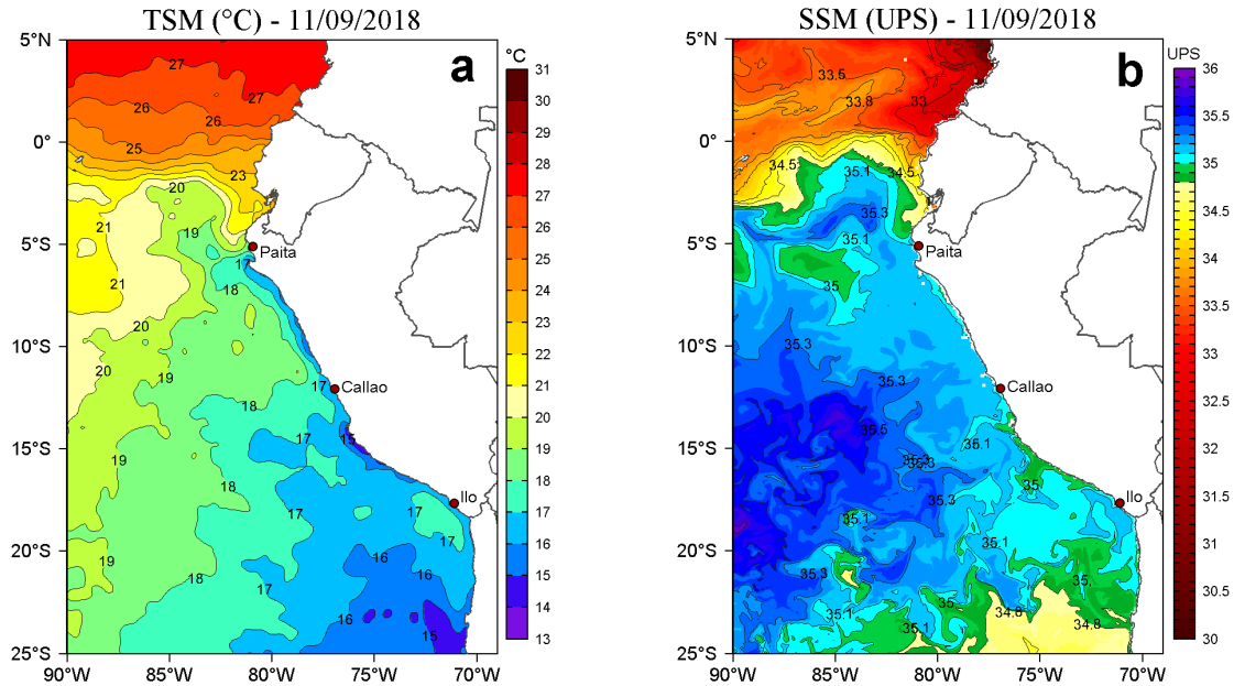
Figura 2. a) Temperatura superficial del mar TSM ( ^{\circ}\text{C} ) y b) Salinidad superficial del mar SSM (UPS) para el 11 de setiembre de 2018. Datos: OSTIA-UKMO-L4-GLOB-v2.0 (UK Met Office, 2012; Donlon et al, 2012) disponible en https://podaac.jpl.nasa.gov/dataset/OSTIA-UKMO-L4-GLOB-v2.0 para (a) y Hybrid Coordinate Ocean Model (HYCOM; Halliwell et al., 1998; 2000; Bleck, 2001) para (b). Procesamiento: LHF/AFIOF/DGIOCC/IMARPE.
