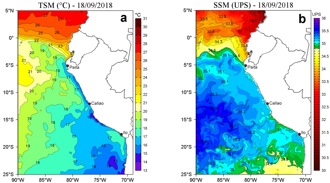
Figura 2. a) Temperatura superficial del mar TSM ( ^{\circ}\text{C} ) y b) Salinidad superficial del mar SSM (UPS) para el 18 de setiembre de 2018. Datos: OSTIA-UKMO-L4-GLOB-v2.0 (UK Met Office, 2012; Donlon et al, 2012) disponible en https://podaac.jpl.nasa.gov/dataset/OSTIA-UKMO-L4-GLOB-v2.0 ) para (a) y Hybrid Coordinate Ocean Model (HYCOM; Halliwell et al., 1998; 2000; Bleck, 2001) para (b). Procesamiento: LHF/AFIOF/DGIOCC/IMARPE.
