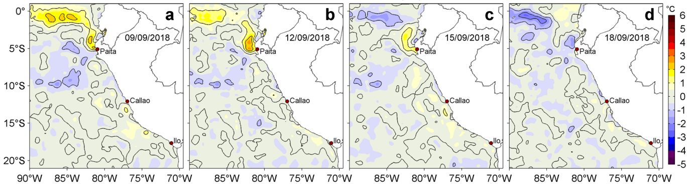
Figura 3. Anomalías de la temperatura superficial del mar TSM ( ^{\circ}\text{C} ) para los días: a) 09, b) 12, c) 15 y d) 18 de setiembre de 2018. Las anomalías se calcularon respecto de la climatología para el periodo 2007-2016. Datos: OSTIA-UKMO-L4-GLOB-v2.0 (UK Met Office, 2012; Donlon et al, 2012). Procesamiento: LHF/AFIOF/DGIOCC/IMARPE.
