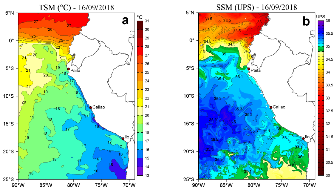
Figura 2. a) Temperatura superficial del mar TSM ( ^{\circ}\text{C} ) y b) Salinidad superficial del mar SSM (UPS) para el 16 de setiembre de 2018. Datos: OSTIA-UKMO-L4-GLOB-v2.0 (UK Met Office, 2012; Donlon et al, 2012) disponible en https://podaac.jpl.nasa.gov/dataset/OSTIA-UKMO-L4-GLOB-v2.0 ) para (a) y Hybrid Coordinate Ocean Model (HYCOM; Halliwell et al., 1998; 2000; Bleck, 2001) para (b). Procesamiento: LHF/AFIOF/DGIOCC/IMARPE.
