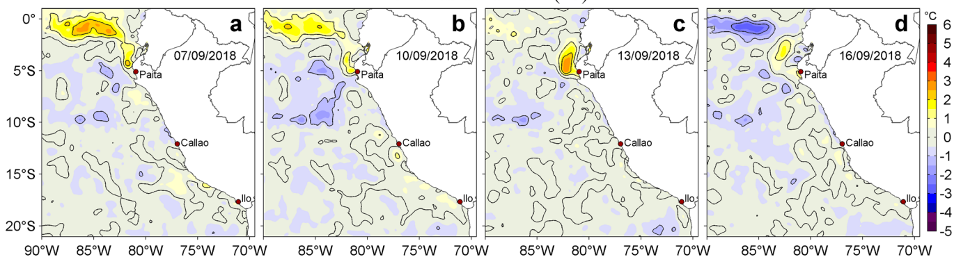
Figura 3. Anomalías de la temperatura superficial del mar TSM ( ^{\circ}\text{C} ) para los días: a) 07, b) 10, c) 13 y d) 16 de setiembre de 2018. Las anomalías se calcularon respecto de la climatología para el periodo 2007-2016. Datos: OSTIA-UKMO-L4-GLOB-v2.0 (UK Met Office, 2012; Donlon et al, 2012). Procesamiento: LHF/AFIOF/DGIOCC/IMARPE.
