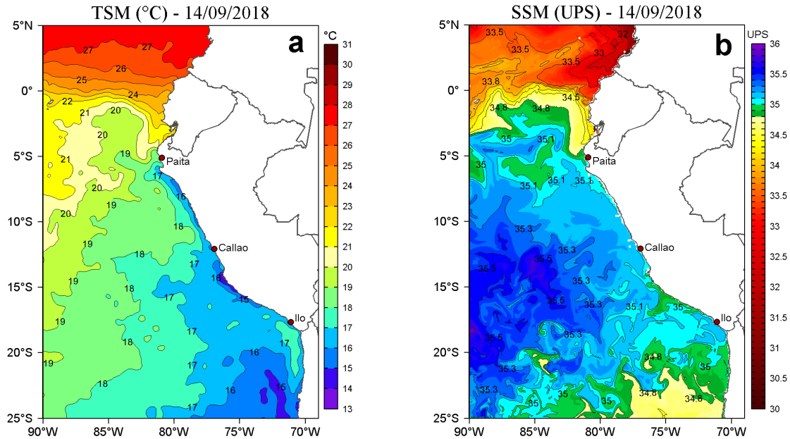
Figura 2. a) Temperatura superficial del mar TSM ( ^{\circ}\text{C} ) y b) Salinidad superficial del mar SSM (UPS) para el 14 de setiembre de 2018. Datos: OSTIA-UKMO-L4-GLOB-v2.0 (UK Met Office, 2012; Donlon et al, 2012) disponible en https://podaac.jpl.nasa.gov/dataset/OSTIA-UKMO-L4-GLOB-v2.0 ) para (a) y Hybrid Coordinate Ocean Model (HYCOM; Halliwell et al., 1998; 2000; Bleck, 2001) para (b). Procesamiento: LHF/AFIOF/DGIOCC/IMARPE.
