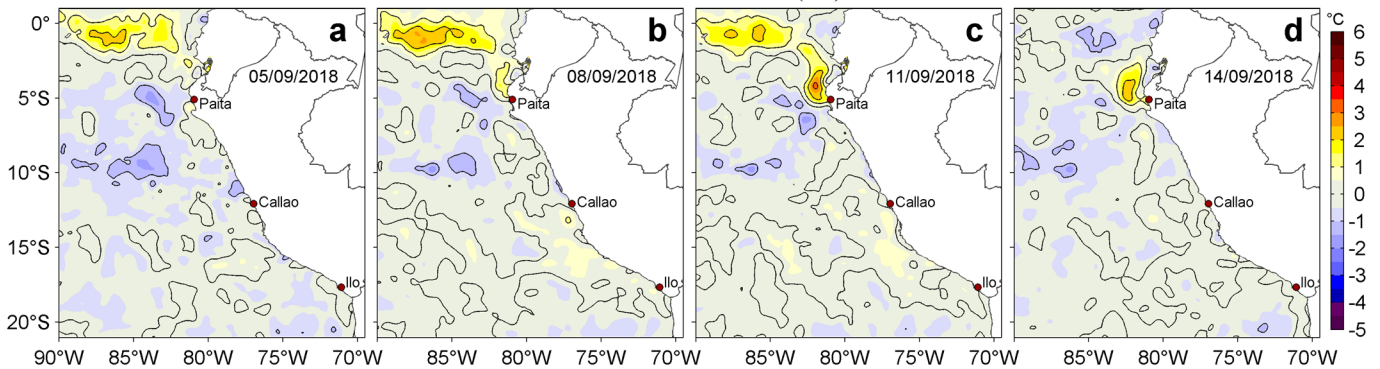
Figura 3. Anomalías de la temperatura superficial del mar TSM ( ^{\circ}\text{C} ) para los días: a) 05, b) 08, c) 11 y d) 14 de setiembre de 2018. Las anomalías se calcularon respecto de la climatología para el periodo 2007-2016. Datos: OSTIA-UKMO-L4-GLOB-v2.0 (UK Met Office, 2012; Donlon et al, 2012). Procesamiento: LHF/AFIOF/DGIOCC/IMARPE.
