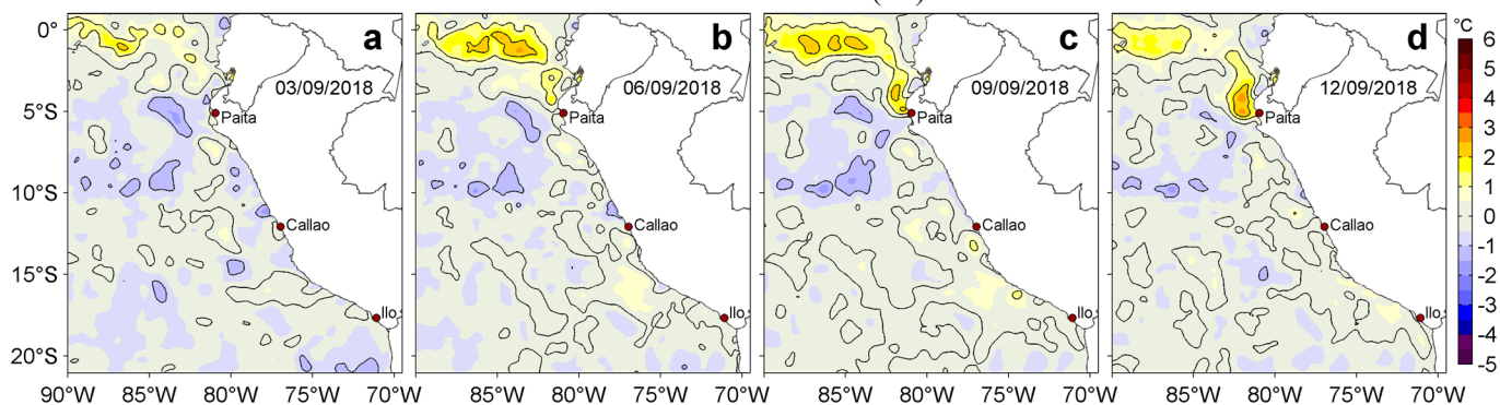
Figura 3. Anomalías de la temperatura superficial del mar TSM ( ^{\circ}\text{C} ) para los días: a) 03, b) 06, c) 09 y d) 12 de setiembre de 2018. Las anomalías se calcularon respecto de la climatología para el periodo 2007-2016. Datos: OSTIA-UKMO-L4-GLOB-v2.0 (UK Met Office, 2012; Donlon et al, 2012). Procesamiento: LHF/AFIOF/DGIOCC/IMARPE.
