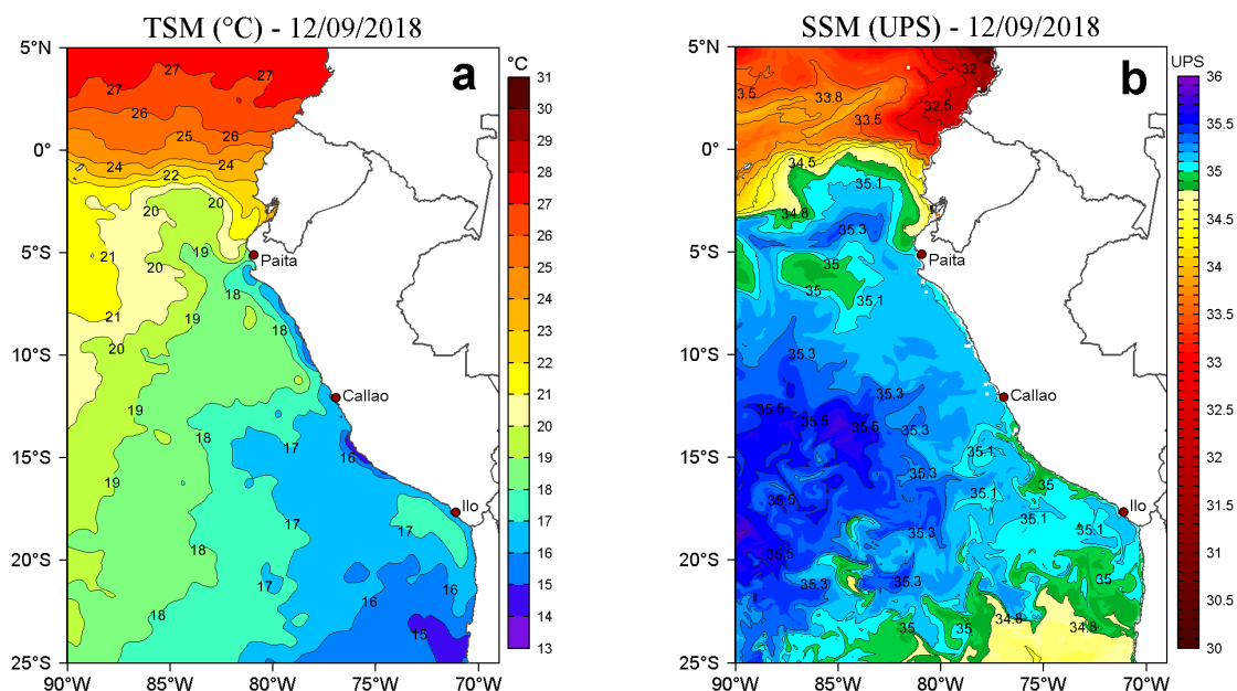
Figura 2. a) Temperatura superficial del mar TSM ( ^{\circ}\text{C} ) y b) Salinidad superficial del mar SSM (UPS) para el 12 de setiembre de 2018. Datos: OSTIA-UKMO-L4-GLOB-v2.0 (UK Met Office, 2012; Donlon et al, 2012) disponible en https://podaac.jpl.nasa.gov/dataset/OSTIA-UKMO-L4-GLOB-v2.0 para (a) y Hybrid Coordinate Ocean Model (HYCOM; Halliwell et al., 1998; 2000; Bleck, 2001) para (b). Procesamiento: LHF/AFIOF/DGIOCC/IMARPE.
