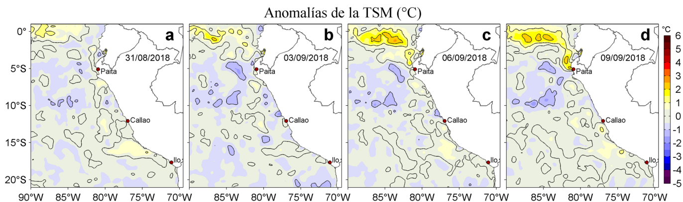
Figura 3. Anomalías de la temperatura superficial del mar TSM ( ^{\circ}\text{C} ) para los días: a) 31 de agosto, b) 03, c) 06 y d) 09 de setiembre de 2018. Las anomalías se calcularon respecto de la climatología para el periodo 2007-2016. Datos: OSTIA-UKMO-L4-GLOB-v2.0 (UK Met Office, 2012; Donlon et al, 2012). Procesamiento: LHF/AFIOF/DGIOCC/IMARPE.
