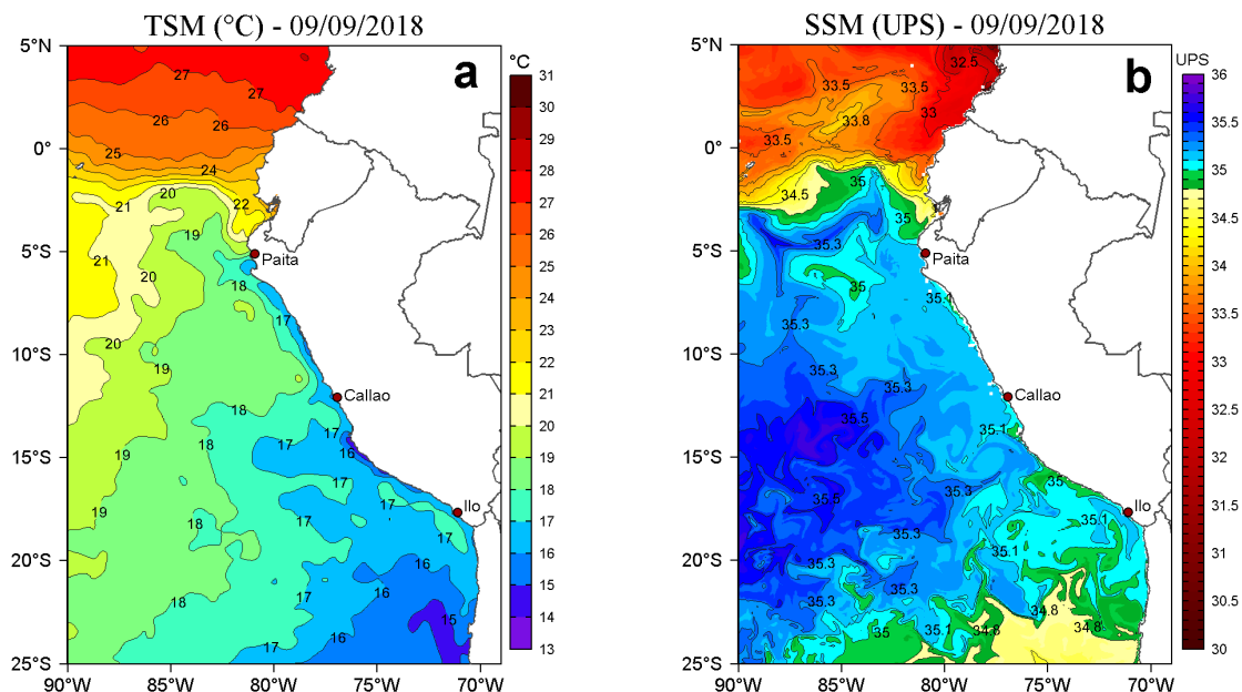
Figura 2. a) Temperatura superficial del mar TSM ( ^{\circ}\text{C} ) y b) Salinidad superficial del mar SSM (UPS) para el 09 de setiembre de 2018. Datos: OSTIA-UKMO-L4-GLOB-v2.0 (UK Met Office, 2012; Donlon et al, 2012) disponible en https://podaac.jpl.nasa.gov/dataset/OSTIA-UKMO-L4-GLOB-v2.0 ) para (a) y Hybrid Coordinate Ocean Model (HYCOM; Halliwell et al., 1998; 2000; Bleck, 2001) para (b). Procesamiento: LHF/AFIOF/DGIOCC/IMARPE.
