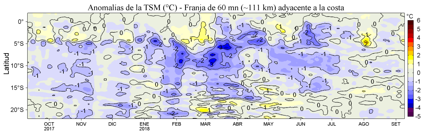
Figura 4. Variación promedio de las anomalías de la temperatura superficial del mar TSM ( ^{\circ}\text{C} ) para una franja de 60 mn ( \sim 111 km) adyacente al litoral peruano para los últimos doce meses al 09 de setiembre de 2018. Datos: OSTIA-UKMO-L4-GLOB-v2.0 (UK Met Office, 2012; Donlon et al, 2012) disponible en https://podaac.jpl.nasa.gov/dataset/OSTIA-UKMO-L4-GLOB-v2.0 ). Las anomalías se calcularon con respecto al periodo 2007-2016. Procesamiento: LHF/AFIOF/DGIOCC/IMARPE.
