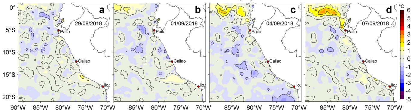
Figura 3. Anomalías de la temperatura superficial del mar TSM ( ^{\circ}\text{C} ) para los días: a) 29 de agosto, b) 01, c) 04 y d) 07 de setiembre de 2018. Las anomalías se calcularon respecto de la climatología para el periodo 2007-2016. Datos: OSTIA-UKMO-L4-GLOB-v2.0 (UK Met Office, 2012; Donlon et al, 2012). Procesamiento: LHF/AFIOF/DGIOCC/IMARPE.
