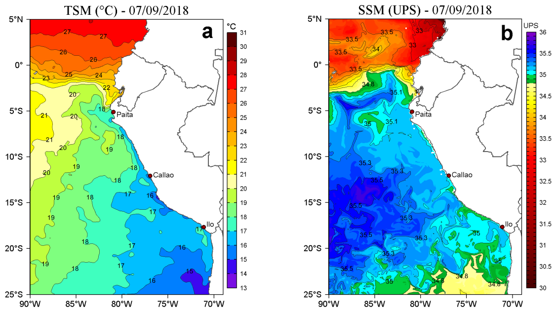
Figura 2. a) Temperatura superficial del mar TSM ( ^{\circ}\text{C} ) y b) Salinidad superficial del mar SSM (UPS) para el 07 de setiembre de 2018. Datos: OSTIA-UKMO-L4-GLOB-v2.0 (UK Met Office, 2012; Donlon et al, 2012) disponible en https://podaac.jpl.nasa.gov/dataset/OSTIA-UKMO-L4-GLOB-v2.0 ) para (a) y Hybrid Coordinate Ocean Model (HYCOM; Halliwell et al., 1998; 2000; Bleck, 2001) para (b). Procesamiento: LHF/AFIOF/DGIOCC/IMARPE.
