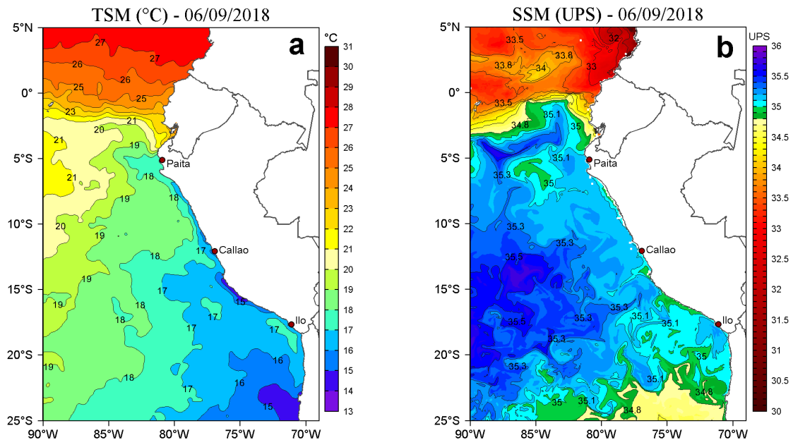
Figura 2. a) Temperatura superficial del mar TSM ( ^{\circ}\text{C} ) y b) Salinidad superficial del mar SSM (UPS) para el 06 de setiembre de 2018. Datos: OSTIA-UKMO-L4-GLOB-v2.0 (UK Met Office, 2012; Donlon et al, 2012) disponible en https://podaac.jpl.nasa.gov/dataset/OSTIA-UKMO-L4-GLOB-v2.0 ) para (a) y Hybrid Coordinate Ocean Model (HYCOM; Halliwell et al., 1998; 2000; Bleck, 2001) para (b). Procesamiento: LHF/AFIOF/DGIOCC/IMARPE.
