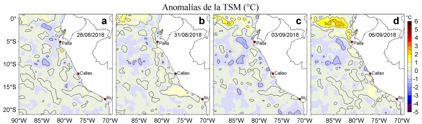
Figura 3. Anomalías de la temperatura superficial del mar TSM ( ^{\circ}\text{C} ) para los días: a) 28 y b) 31 de agosto, c) 03 y d) 06 de setiembre de 2018. Las anomalías se calcularon respecto de la climatología para el periodo 2007-2016. Datos: OSTIA-UKMO-L4-GLOB-v2.0 (UK Met Office, 2012; Donlon et al, 2012). Procesamiento: LHF/AFIOF/DGIOCC/IMARPE.
