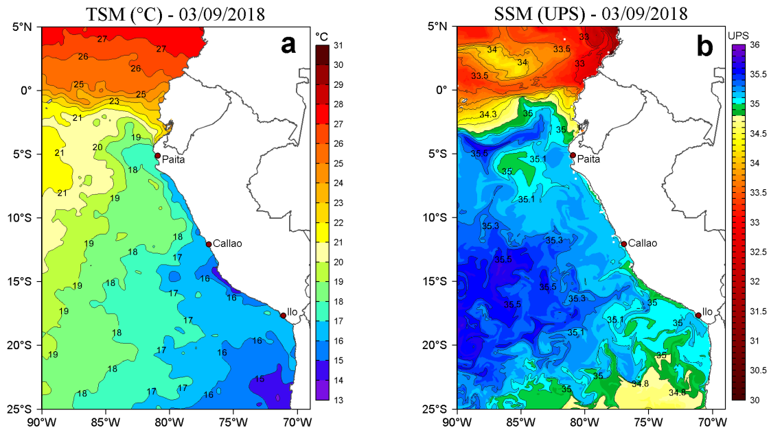
Figura 2. a) Temperatura superficial del mar TSM ( ^{\circ}\text{C} ) y b) Salinidad superficial del mar SSM (UPS) para el 03 de setiembre de 2018. Datos: OSTIA-UKMO-L4-GLOB-v2.0 (UK Met Office, 2012; Donlon et al, 2012) disponible en https://podaac.jpl.nasa.gov/dataset/OSTIA-UKMO-L4-GLOB-v2.0 ) para (a) y Hybrid Coordinate Ocean Model (HYCOM; Halliwell et al., 1998; 2000; Bleck, 2001) para (b). Procesamiento: LHF/AFIOF/DGIOCC/IMARPE.
