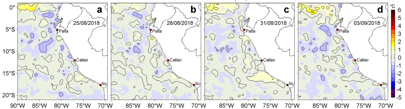
Figura 3. Anomalías de la temperatura superficial del mar TSM ( ^{\circ}\text{C} ) para los días: a) 25, b) 28 y c) 31 de agosto y d) 03 de setiembre de 2018. Las anomalías se calcularon respecto de la climatología para el periodo 2007-2016. Datos: OSTIA-UKMO-L4-GLOB-v2.0 (UK Met Office, 2012; Donlon et al, 2012). Procesamiento: LHF/AFIOF/DGIOCC/IMARPE.
