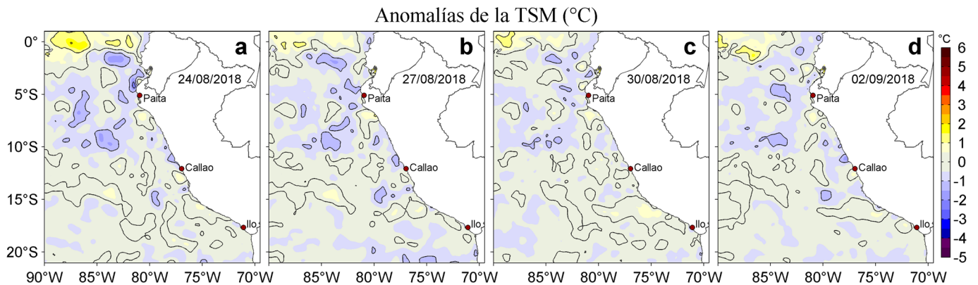
Figura 3. Anomalías de la temperatura superficial del mar TSM ( ^{\circ}\text{C} ) para los días: a) 24, b) 27 y c) 30 de agosto y d) 02 de setiembre de 2018. Las anomalías se calcularon respecto de la climatología para el periodo 2007-2016. Datos: OSTIA-UKMO-L4-GLOB-v2.0 (UK Met Office, 2012; Donlon et al, 2012). Procesamiento: LHF/AFIOF/DGIOCC/IMARPE.
