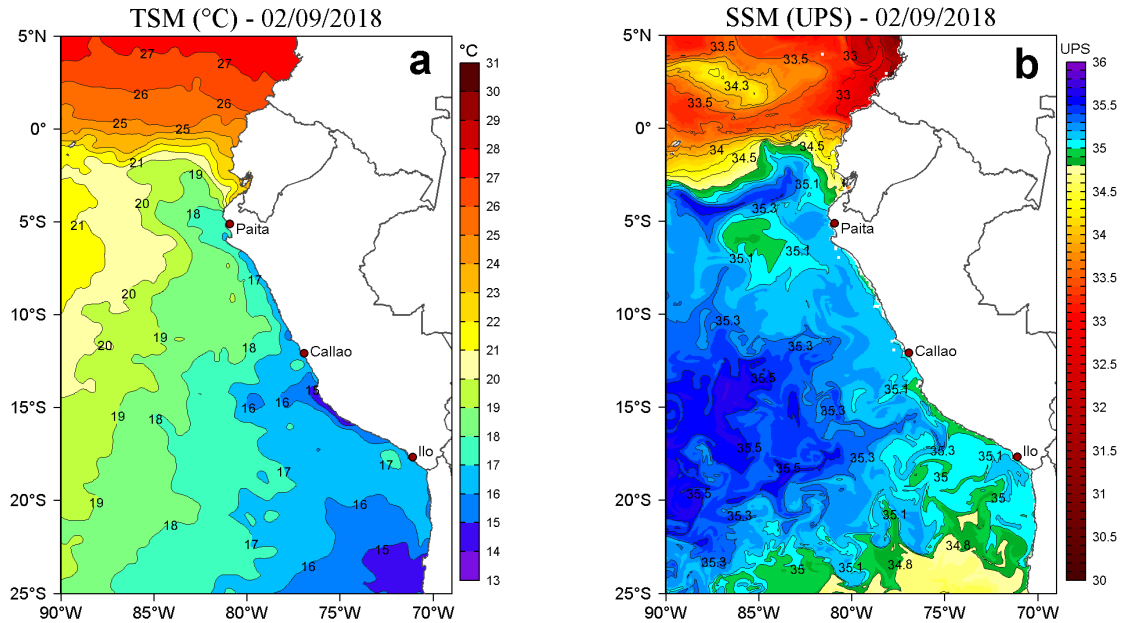
Figura 2. a) Temperatura superficial del mar TSM ( ^{\circ}\text{C} ) y b) Salinidad superficial del mar SSM (UPS) para el 02 de setiembre de 2018. Datos: OSTIA-UKMO-L4-GLOB-v2.0 (UK Met Office, 2012; Donlon et al, 2012) disponible en https://podaac.jpl.nasa.gov/dataset/OSTIA-UKMO-L4-GLOB-v2.0 ) para (a) y Hybrid Coordinate Ocean Model (HYCOM; Halliwell et al., 1998; 2000; Bleck, 2001) para (b). Procesamiento: LHF/AFIOF/DGIOCC/IMARPE.
