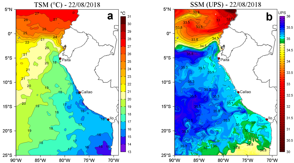
Figura 2. a) Temperatura superficial del mar TSM ( ^{\circ}\text{C} ) y b) Salinidad superficial del mar SSM (UPS) para el 22 de agosto de 2018. Datos: OSTIA-UKMO-L4-GLOB-v2.0 (UK Met Office, 2012; Donlon et al, 2012) disponible en https://podaac.jpl.nasa.gov/dataset/OSTIA-UKMO-L4-GLOB-v2.0 para (a) y Hybrid Coordinate Ocean Model (HYCOM; Halliwell et al., 1998; 2000; Bleck, 2001) para (b). Procesamiento: LHF/AFIOF/DGIOCC/IMARPE.
