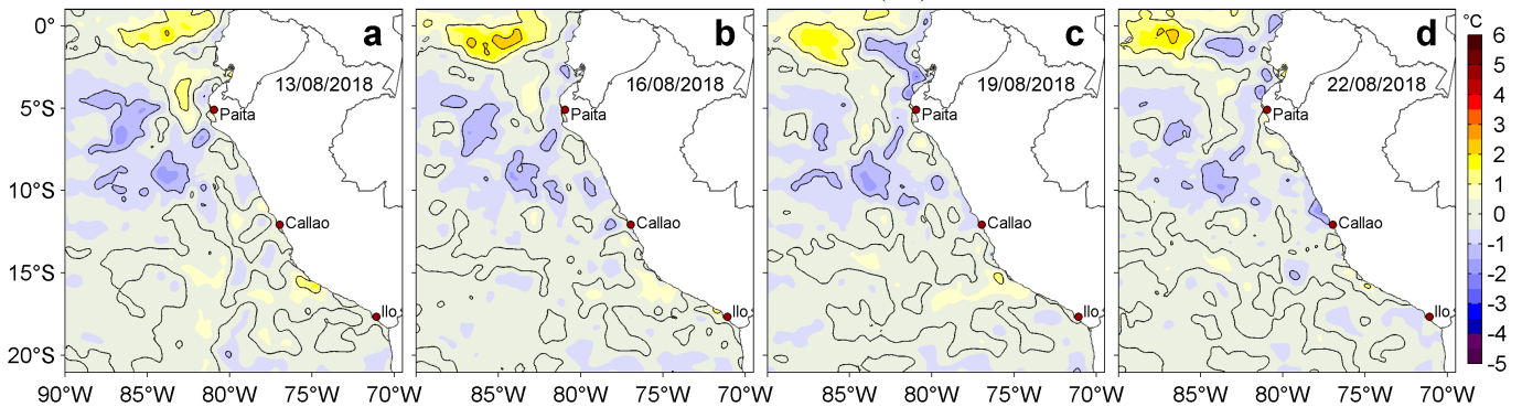
Figura 3. Anomalías de la temperatura superficial del mar TSM ( ^{\circ}\text{C} ) para los días: a) 13, b) 16, c) 19 y d) 22 de agosto de 2018. Las anomalías se calcularon respecto de la climatología para el periodo 2007-2016. Datos: OSTIA-UKMO-L4-GLOB-v2.0 (UK Met Office, 2012; Donlon et al, 2012). Procesamiento: LHF/AFIOF/DGIOCC/IMARPE.
