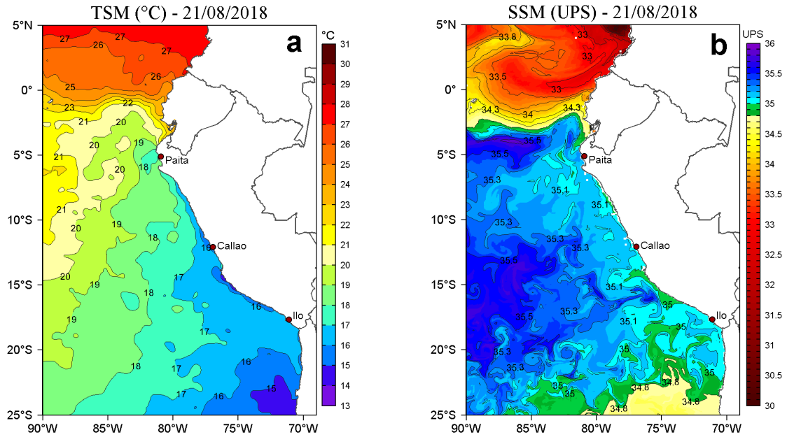
Figura 2. a) Temperatura superficial del mar TSM ( ^{\circ}\text{C} ) y b) Salinidad superficial del mar SSM (UPS) para el 21 de agosto de 2018. Datos: OSTIA-UKMO-L4-GLOB-v2.0 (UK Met Office, 2012; Donlon et al, 2012) disponible en https://podaac.jpl.nasa.gov/dataset/OSTIA-UKMO-L4-GLOB-v2.0 para (a) y Hybrid Coordinate Ocean Model (HYCOM; Halliwell et al., 1998; 2000; Bleck, 2001) para (b). Procesamiento: LHF/AFIOF/DGIOCC/IMARPE.
