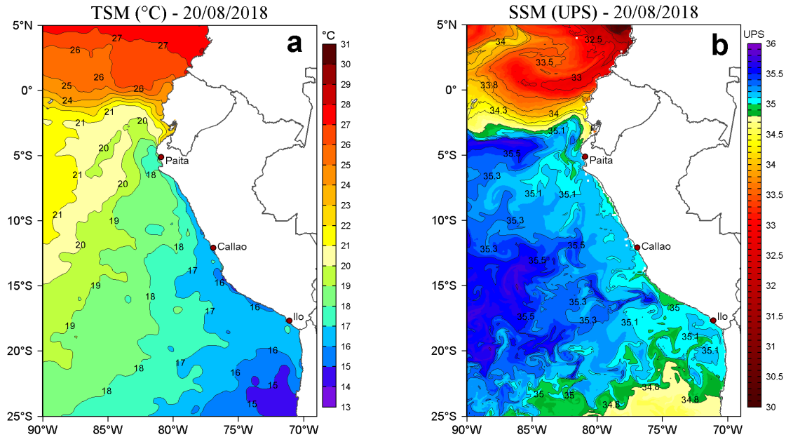
Figura 2. a) Temperatura superficial del mar TSM ( ^{\circ}\text{C} ) y b) Salinidad superficial del mar SSM (UPS) para el 20 de agosto de 2018. Datos: OSTIA-UKMO-L4-GLOB-v2.0 (UK Met Office, 2012; Donlon et al, 2012) disponible en https://podaac.jpl.nasa.gov/dataset/OSTIA-UKMO-L4-GLOB-v2.0 para (a) y Hybrid Coordinate Ocean Model (HYCOM; Halliwell et al., 1998; 2000; Bleck, 2001) para (b). Procesamiento: LHF/AFIOF/DGIOCC/IMARPE.
