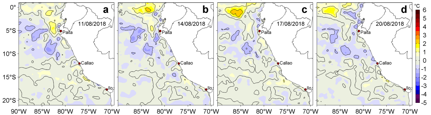
Figura 3. Anomalías de la temperatura superficial del mar TSM ( ^{\circ}\text{C} ) para los días: a) 11, b) 14, c) 17 y d) 20 de agosto de 2018. Las anomalías se calcularon respecto de la climatología para el periodo 2007-2016. Datos: OSTIA-UKMO-L4-GLOB-v2.0 (UK Met Office, 2012; Donlon et al, 2012). Procesamiento: LHF/AFIOF/DGIOCC/IMARPE.
