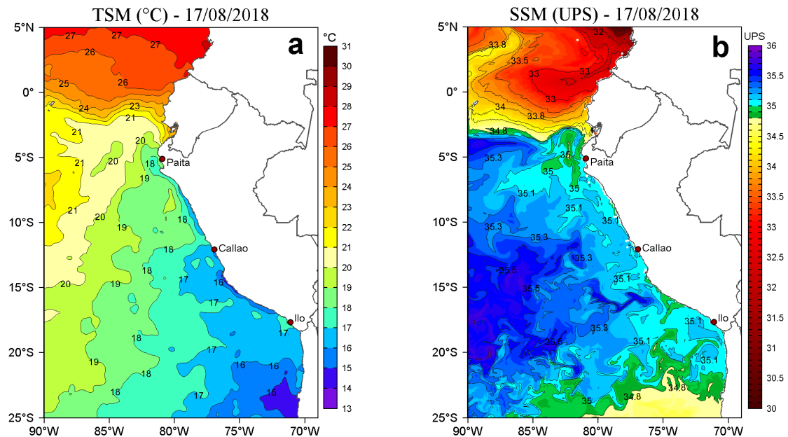
Figura 2. a) Temperatura superficial del mar TSM ( ^{\circ}\text{C} ) y b) Salinidad superficial del mar SSM (UPS) para el 17 de agosto de 2018. Datos: OSTIA-UKMO-L4-GLOB-v2.0 (UK Met Office, 2012; Donlon et al, 2012) disponible en https://podaac.jpl.nasa.gov/dataset/OSTIA-UKMO-L4-GLOB-v2.0 para (a) y Hybrid Coordinate Ocean Model (HYCOM; Halliwell et al., 1998; 2000; Bleck, 2001) para (b). Procesamiento: LHF/AFIOF/DGIOCC/IMARPE.
