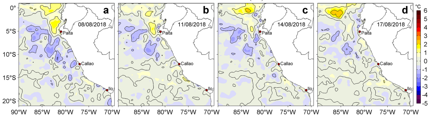
Figura 3. Anomalías de la temperatura superficial del mar TSM ( ^{\circ}\text{C} ) para los días: a) 08, b) 11, c) 14 y d) 17 de agosto de 2018. Las anomalías se calcularon respecto de la climatología para el periodo 2007-2016. Datos: OSTIA-UKMO-L4-GLOB-v2.0 (UK Met Office, 2012; Donlon et al, 2012). Procesamiento: LHF/AFIOF/DGIOCC/IMARPE.
