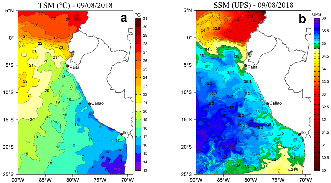
Figura 2. a) Temperatura superficial del mar TSM ( ^{\circ}\text{C} ) y b) Salinidad superficial del mar SSM (UPS) para el 09 de agosto de 2018. Datos: OSTIA-UKMO-L4-GLOB-v2.0 (UK Met Office, 2012; Donlon et al, 2012) disponible en https://podaac.jpl.nasa.gov/dataset/OSTIA-UKMO-L4-GLOB-v2.0 para (a) y Hybrid Coordinate Ocean Model (HYCOM; Halliwell et al., 1998; 2000; Bleck, 2001) para (b). Procesamiento: LHF/AFIOF/DGIOCC/IMARPE.
