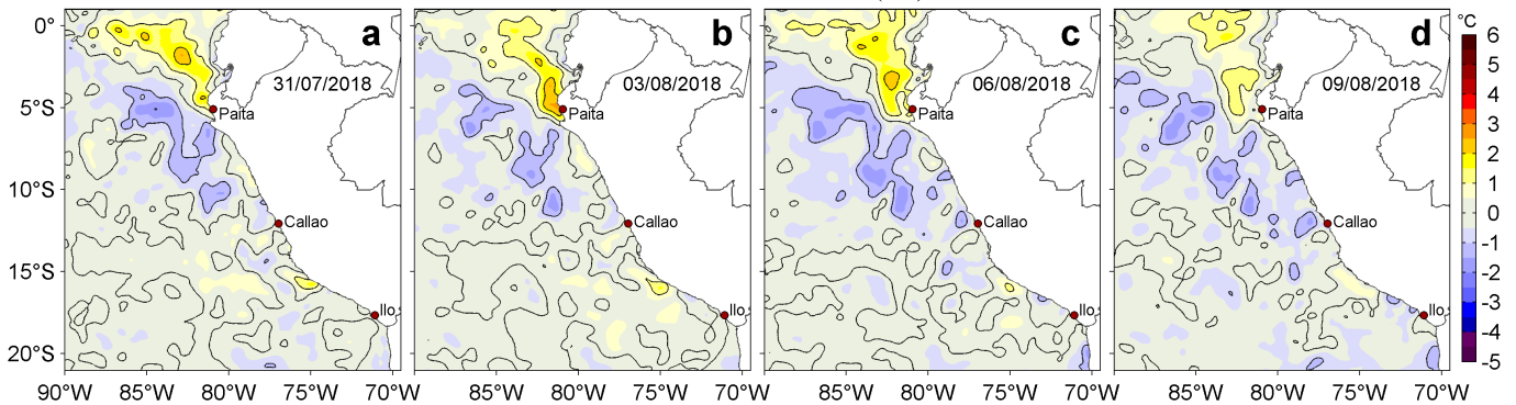
Figura 3. Anomalías de la temperatura superficial del mar TSM ( ^{\circ}\text{C} ) para los días: a) 31 de julio y b) 03, c) 06 y d) 09 de agosto de 2018. Las anomalías se calcularon respecto de la climatología para el periodo 2007-2016. Datos: OSTIA-UKMO-L4-GLOB-v2.0 (UK Met Office, 2012; Donlon et al, 2012). Procesamiento: LHF/AFIOF/DGIOCC/IMARPE.
