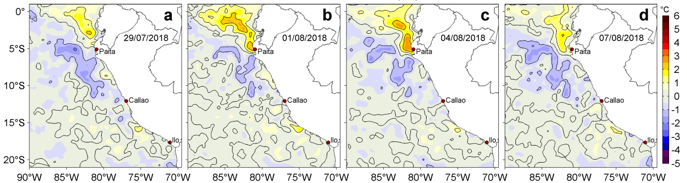
Figura 3. Anomalías de la temperatura superficial del mar TSM ( ^{\circ}\text{C} ) para los días: a) 29 de julio y b) 01, c) 04 y d) 07 de agosto de 2018. Las anomalías se calcularon respecto de la climatología para el periodo 2007-2016. Datos: OSTIA-UKMO-L4-GLOB-v2.0 (UK Met Office, 2012; Donlon et al, 2012). Procesamiento: LHF/AFIOF/DGIOCC/IMARPE.
