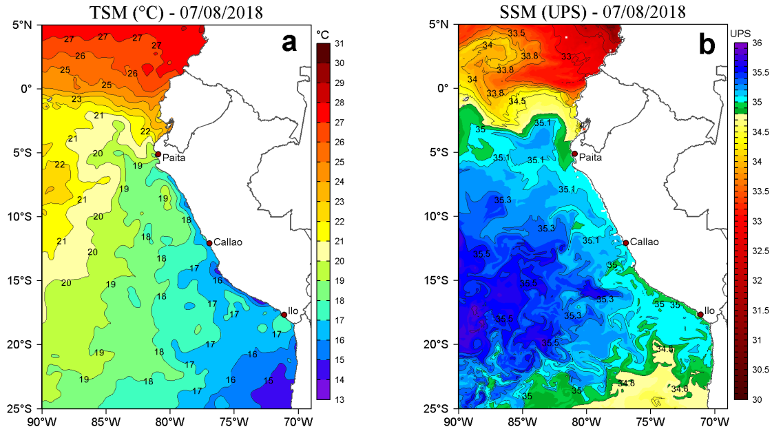
Figura 2. a) Temperatura superficial del mar TSM ( ^{\circ}\text{C} ) y b) Salinidad superficial del mar SSM (UPS) para el 07 de agosto de 2018. Datos: OSTIA-UKMO-L4-GLOB-v2.0 (UK Met Office, 2012; Donlon et al, 2012) disponible en https://podaac.jpl.nasa.gov/dataset/OSTIA-UKMO-L4-GLOB-v2.0 para (a) y Hybrid Coordinate Ocean Model (HYCOM; Halliwell et al., 1998; 2000; Bleck, 2001) para (b). Procesamiento: LHF/AFIOF/DGIOCC/IMARPE.
