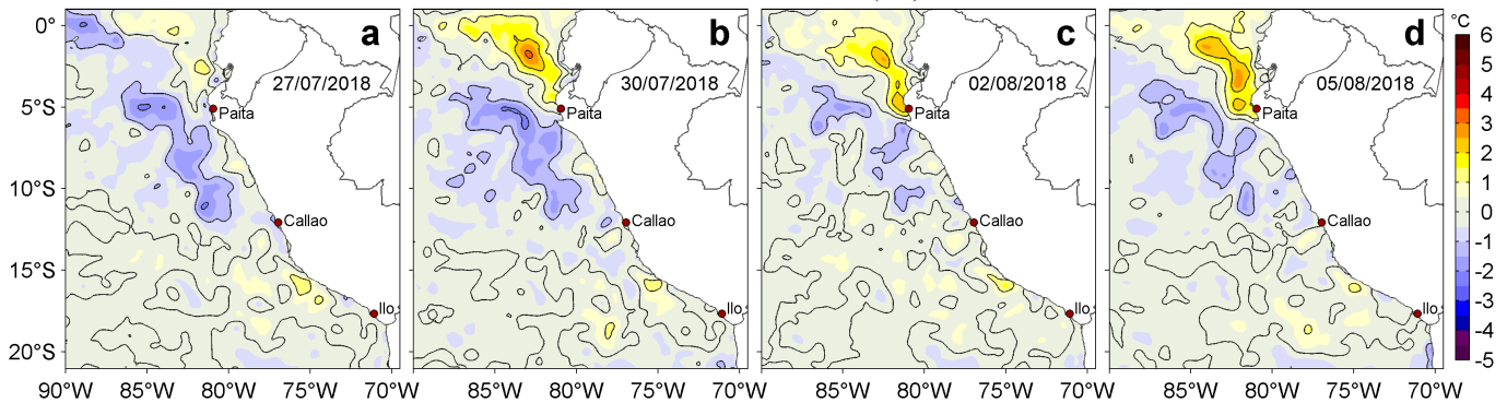
Figura 3. Anomalías de la Temperatura Superficial del Mar (°C) para los días: a) 27 y b) 30 de julio c) 02 y d) 05 de agosto de 2018. Las anomalías se calcularon respecto de la climatología para el periodo 2007-2016. Datos: OSTIA-UKMO-L4-GLOB-v2.0 (UK Met Office, 2012; Donlon et al, 2012). Procesamiento: LHF/AFIOF/DGIOCC/IMARPE.
