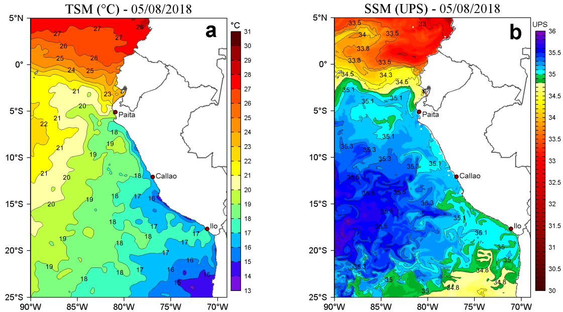
Figura 2. a) Temperatura Superficial del Mar (°C) y b) Salinidad Superficial del Mar (UPS) para el 05 de agosto de 2018. Datos: OSTIA-UKMO-L4-GLOB-v2.0 (UK Met Office, 2012; Donlon et al, 2012) disponible en https://podaac.jpl.nasa.gov/dataset/OSTIA-UKMO-L4-GLOB-v2.0 para (a) y Hybrid Coordinate Ocean Model (HYCOM; Halliwell et al., 1998; 2000; Bleck, 2001) para (b). Procesamiento: LHF/AFIOF/DGIOCC/IMARPE.
