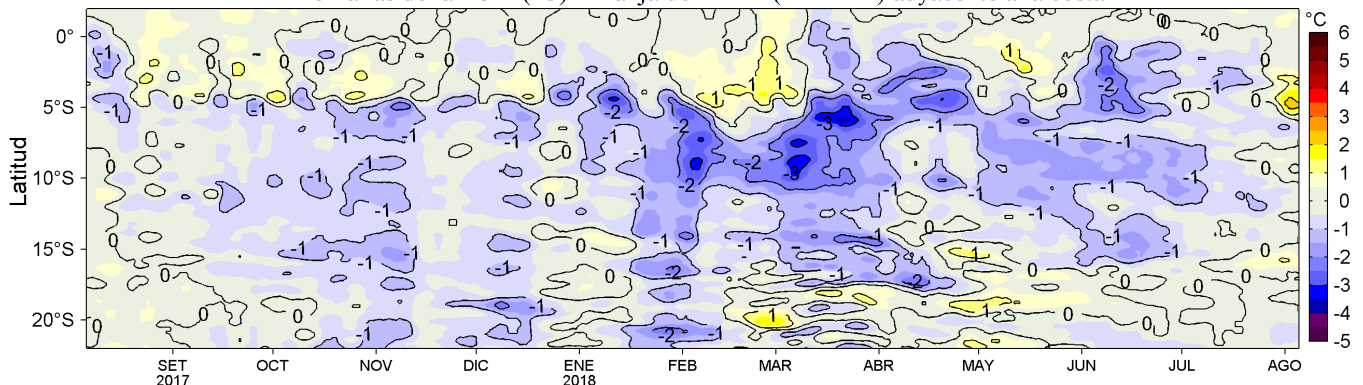
Figura 4. Variación promedio de las anomalías de la Temperatura Superficial del Mar (°C) para una franja de 60 mn (~111 km) adyacente al litoral peruano para los últimos doce meses al 05 de agosto de 2018. Datos: OSTIA-UKMO-L4-GLOB-v2.0 (UK Met Office, 2012; Donlon et al, 2012) disponible en https://podaac.jpl.nasa.gov/dataset/OSTIA-UKMO-L4-GLOB-v2.0 . Las anomalías se calcularon con respecto al periodo 2007-2016. Procesamiento: LHF/AFIOF/DGIOCC/IMARPE.
