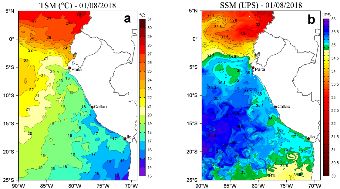
Figura 2. a) Temperatura Superficial del Mar ( ^{\circ}\text{C} ) y b) Salinidad Superficial del Mar (UPS) para el 01 de agosto de 2018. Datos: OSTIA-UKMO-L4-GLOB-v2.0 (UK Met Office, 2012; Donlon et al, 2012) disponible en https://podaac.jpl.nasa.gov/dataset/OSTIA-UKMO-L4-GLOB-v2.0 para (a) y Hybrid Coordinate Ocean Model (HYCOM; Halliwell et al., 1998; 2000; Bleck, 2001) para (b). Procesamiento: LHF/AFIOF/DGIOCC/IMARPE.
