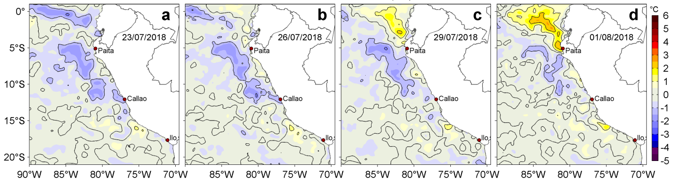
Figura 3. Anomalías de la Temperatura Superficial del Mar ( ^{\circ}\text{C} ) para los días: a) 23, b) 26 y c) 29 de julio y d) 01 de agosto de 2018. Las anomalías se calcularon respecto de la climatología para el periodo 2007-2016. Datos: OSTIA-UKMO-L4-GLOB-v2.0 (UK Met Office, 2012; Donlon et al, 2012). Procesamiento: LHF/AFIOF/DGIOCC/IMARPE.
