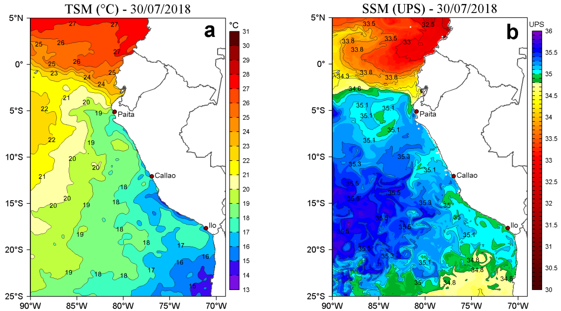
Figura 2. a) Temperatura Superficial del Mar ( ^{\circ}\text{C} ) y b) Salinidad Superficial del Mar (UPS) para el 30 de julio de 2018. Datos: OSTIA-UKMO-L4-GLOB-v2.0 (UK Met Office, 2012; Donlon et al, 2012) disponible en https://podaac.jpl.nasa.gov/dataset/OSTIA-UKMO-L4-GLOB-v2.0 para (a) y Hybrid Coordinate Ocean Model (HYCOM; Halliwell et al., 1998; 2000; Bleck, 2001) para (b). Procesamiento: LHF/AFIOF/DGIOCC/IMARPE.
