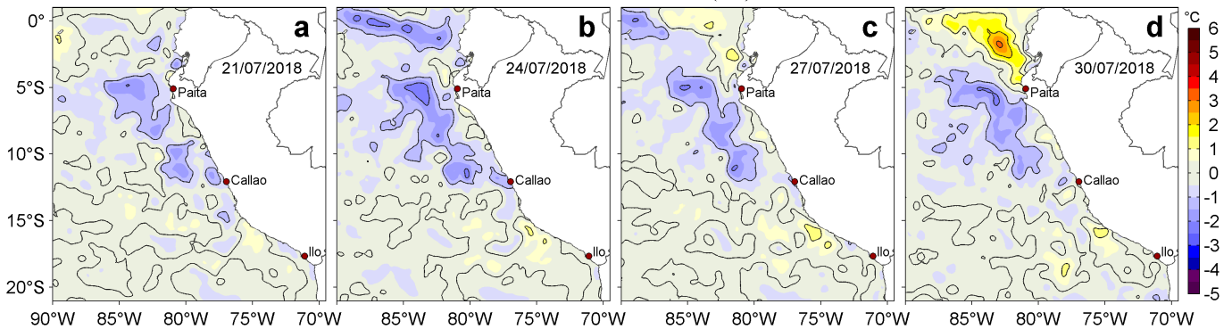
Figura 3. Anomalías de la Temperatura Superficial del Mar ( ^{\circ}\text{C} ) para los días: a) 21, b) 24, c) 27 y d) 30 de julio de 2018. Las anomalías se calcularon respecto de la climatología para el periodo 2007-2016. Datos: OSTIA-UKMO-L4-GLOB-v2.0 (UK Met Office, 2012; Donlon et al, 2012). Procesamiento: LHF/AFIOF/DGIOCC/IMARPE.
