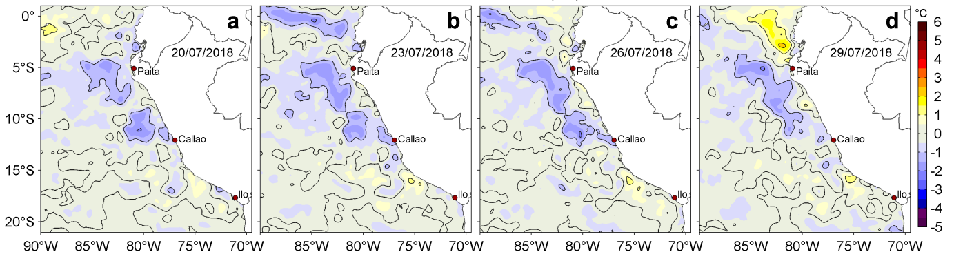
Figura 3. Anomalías de la Temperatura Superficial del Mar ( ^{\circ}\text{C} ) para los días: a) 20, b) 23, c) 26 y d) 29 de julio de 2018. Las anomalías se calcularon respecto de la climatología para el periodo 2007-2016. Datos: OSTIA-UKMO-L4-GLOB-v2.0 (UK Met Office, 2012; Donlon et al, 2012). Procesamiento: LHF/AFIOF/DGIOCC/IMARPE.
