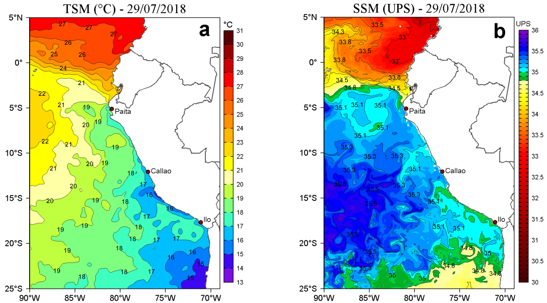
Figura 2. a) Temperatura Superficial del Mar ( ^{\circ}\text{C} ) y b) Salinidad Superficial del Mar (UPS) para el 29 de julio de 2018. Datos: OSTIA-UKMO-L4-GLOB-v2.0 (UK Met Office, 2012; Donlon et al, 2012) disponible en https://podaac.jpl.nasa.gov/dataset/OSTIA-UKMO-L4-GLOB-v2.0 para (a) y Hybrid Coordinate Ocean Model (HYCOM; Halliwell et al., 1998; 2000; Bleck, 2001) para (b). Procesamiento: LHF/AFIOF/DGIOCC/IMARPE.
