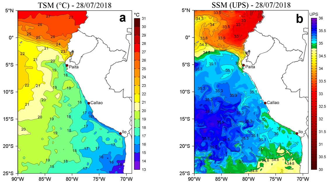
Figura 2. a) Temperatura Superficial del Mar ( ^{\circ}\text{C} ) y b) Salinidad Superficial del Mar (UPS) para el 28 de julio de 2018. Datos: OSTIA-UKMO-L4-GLOB-v2.0 (UK Met Office, 2012; Donlon et al, 2012) disponible en https://podaac.jpl.nasa.gov/dataset/OSTIA-UKMO-L4-GLOB-v2.0 para (a) y Hybrid Coordinate Ocean Model (HYCOM; Halliwell et al., 1998; 2000; Bleck, 2001) para (b). Procesamiento: LHF/AFIOF/DGIOCC/IMARPE.
