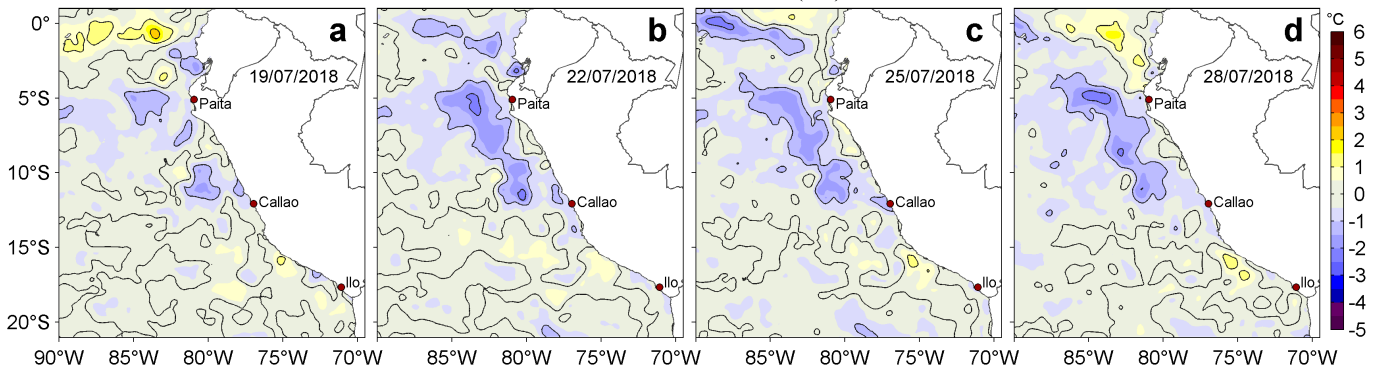
Figura 3. Anomalías de la Temperatura Superficial del Mar ( ^{\circ}\text{C} ) para los días: a) 19, b) 22, c) 25 y d) 28 de julio de 2018. Las anomalías se calcularon respecto de la climatología para el periodo 2007-2016. Datos: OSTIA-UKMO-L4-GLOB-v2.0 (UK Met Office, 2012; Donlon et al, 2012). Procesamiento: LHF/AFIOF/DGIOCC/IMARPE.
