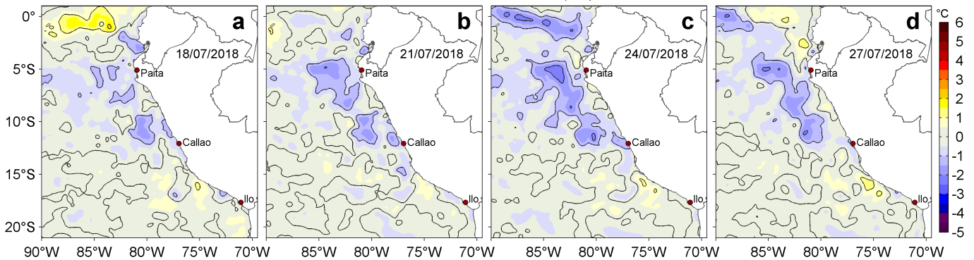
Figura 3. Anomalías de la Temperatura Superficial del Mar (°C) para los días: a) 18, b) 21, c) 24 y d) 27 de julio de 2018. Las anomalías se calcularon respecto de la climatología para el periodo 2007-2016. Datos: OSTIA-UKMO-L4-GLOB-v2.0 (UK Met Office, 2012; Donlon et al, 2012). Procesamiento: LHFM/AFIOF/DGIOCC/IMARPE.
