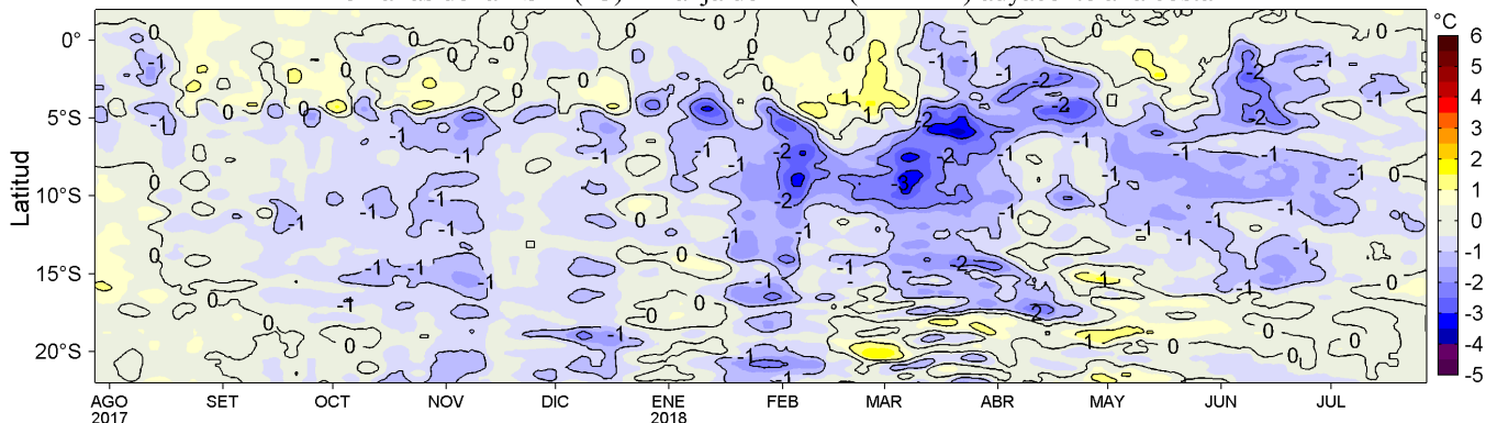
Figura 4. Variación promedio de las anomalías de la Temperatura Superficial del Mar (°C) para una franja de 60 mn (~111 km) adyacente al litoral peruano para los últimos doce meses al 27 de julio de 2018. Datos: OSTIA-UKMO-L4-GLOB-v2.0 (UK Met. Office, 2012; Donlon et al, 2012) disponible en https://podaac.jpl.nasa.gov/dataset/OSTIA-UKMO-L4-GLOB-v2.0 . Las anomalías se calcularon con respecto al periodo 2007-2016. Procesamiento: LHFM/AFIOF/DGIOCC/IMARPE.
