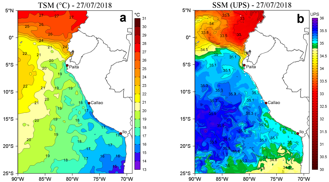
Figura 2. a) Temperatura Superficial del Mar (°C) y b) Salinidad Superficial del Mar (UPS) para el 27 de julio de 2018. Datos: OSTIA-UKMO-L4-GLOB-v2.0 (UK Met Office, 2012; Donlon et al, 2012) disponible en https://podaac.jpl.nasa.gov/dataset/OSTIA-UKMO-L4-GLOB-v2.0 para (a) y Hybrid Coordinate Ocean Model (HYCOM; Halliwell et al., 1998; 2000; Bleck, 2001) para (b). Procesamiento: LHFM/AFIOF/DGIOCC/IMARPE.
