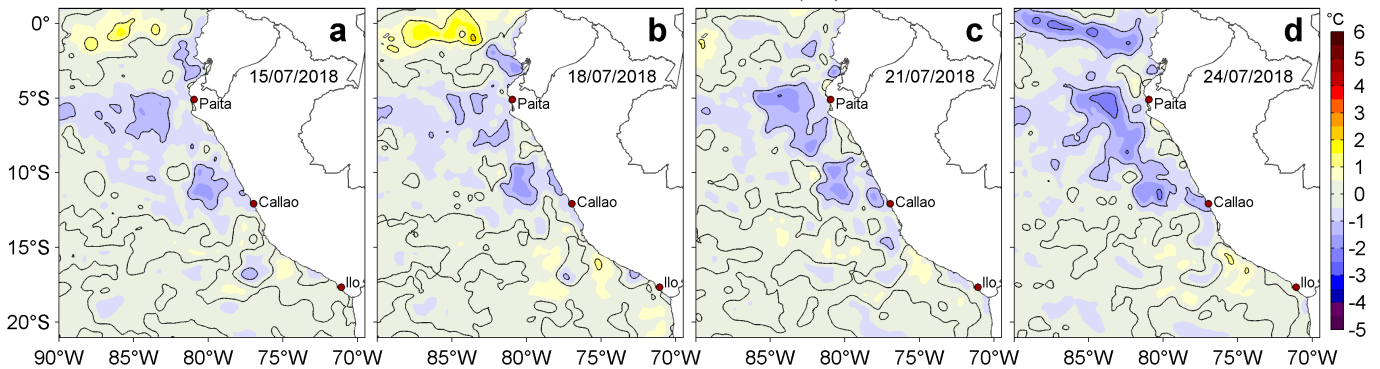
Figura 3. Anomalías de la Temperatura Superficial del Mar ( ^{\circ}\text{C} ) para los días: a) 15, b) 18, c) 21 y d) 24 de julio de 2018. Las anomalías se calcularon respecto de la climatología para el periodo 2007-2016. Datos: OSTIA-UKMO-L4-GLOB-v2.0 (UK Met Office, 2012; Donlon et al, 2012). Procesamiento: LHF/AFIOF/DGIOCC/IMARPE.
