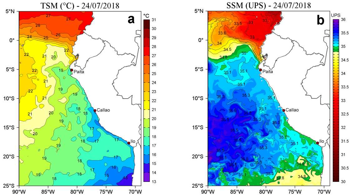
Figura 2. a) Temperatura Superficial del Mar ( ^{\circ}\text{C} ) y b) Salinidad Superficial del Mar (UPS) para el 24 de julio de 2018. Datos: OSTIA-UKMO-L4-GLOB-v2.0 (UK Met Office, 2012; Donlon et al, 2012) disponible en https://podaac.jpl.nasa.gov/dataset/OSTIA-UKMO-L4-GLOB-v2.0 para (a) y Hybrid Coordinate Ocean Model (HYCOM; Halliwell et al., 1998; 2000; Bleck, 2001) para (b). Procesamiento: LHF/AFIOF/DGIOCC/IMARPE.
