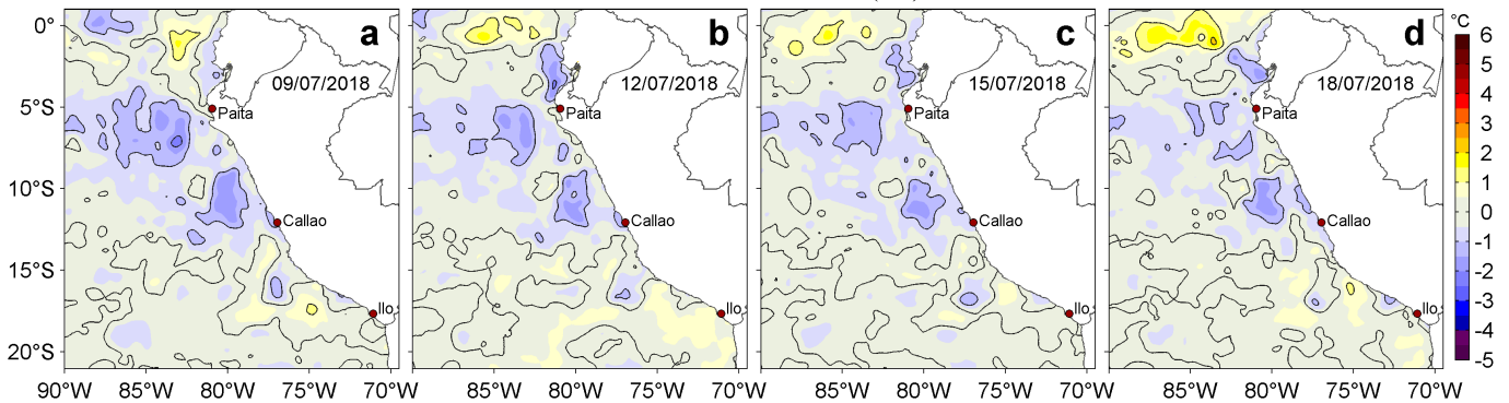
Figura 3. Anomalías de la Temperatura Superficial del Mar ( ^{\circ}\text{C} ) para los días: a) 09, b) 12, c) 15 y d) 18 de julio de 2018. Las anomalías se calcularon respecto de la climatología para el periodo 2007-2016. Datos: OSTIA-UKMO-L4-GLOB-v2.0 (UK Met Office, 2012; Donlon et al, 2012). Procesamiento: LHFM/AFIOF/DGIOCC/IMARPE.
