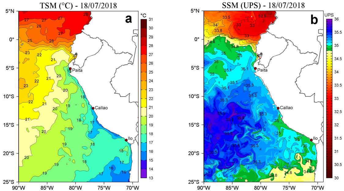
Figura 2. a) Temperatura Superficial del Mar ( ^{\circ}\text{C} ) y b) Salinidad Superficial del Mar (UPS) para el 18 de julio de 2018. Datos: OSTIA-UKMO-L4-GLOB-v2.0 (UK Met Office, 2012; Donlon et al, 2012) disponible en https://podaac.jpl.nasa.gov/dataset/OSTIA-UKMO-L4-GLOB-v2.0 para (a) y Hybrid Coordinate Ocean Model (HYCOM; Halliwell et al., 1998; 2000; Bleck, 2001) para (b). Procesamiento: LHFM/AFIOF/DGIOCC/IMARPE.
