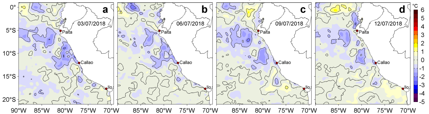
Figura 3. Anomalías de la Temperatura Superficial del Mar ( ^{\circ}\text{C} ) para los días: a) 03, b) 06, c) 09 y d) 12 de julio de 2018. Las anomalías se calcularon respecto de la climatología para el periodo 2007-2016. Datos: OSTIA-UKMO-L4-GLOB-v2.0 (UK Met Office, 2012; Donlon et al, 2012). Procesamiento: LHFM/AFIOF/DGIOCC/IMARPE.
