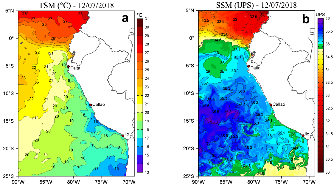
Figura 2. a) Temperatura Superficial del Mar ( ^{\circ}\text{C} ) y b) Salinidad Superficial del Mar (UPS) para el 12 de julio de 2018. Datos: OSTIA-UKMO-L4-GLOB-v2.0 (UK Met Office, 2012; Donlon et al, 2012) disponible en https://podaac.jpl.nasa.gov/dataset/OSTIA-UKMO-L4-GLOB-v2.0 para (a) y Hybrid Coordinate Ocean Model (HYCOM; Halliwell et al., 1998; 2000; Bleck, 2001) para (b). Procesamiento: LHFM/AFIOF/DGIOCC/IMARPE.
