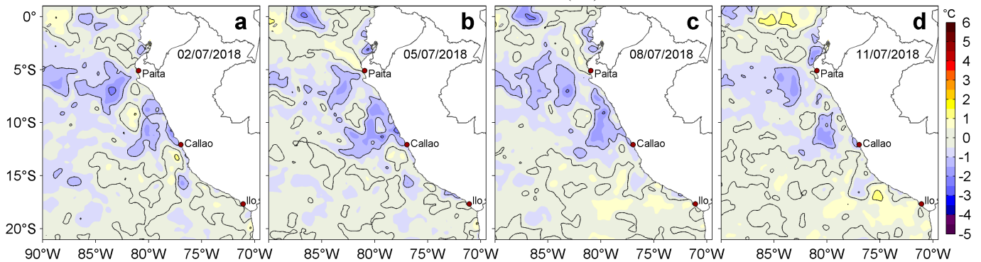
Figura 3. Anomalías de la Temperatura Superficial del Mar ( ^{\circ}\text{C} ) para los días: a) 02, b) 05, c) 08 y d) 11 de julio de 2018. Las anomalías se calcularon respecto de la climatología para el periodo 2007-2016. Datos: OSTIA-UKMO-L4-GLOB-v2.0 (UK Met Office, 2012; Donlon et al, 2012). Procesamiento: LHFM/AFIOF/DGIOCC/IMARPE.
