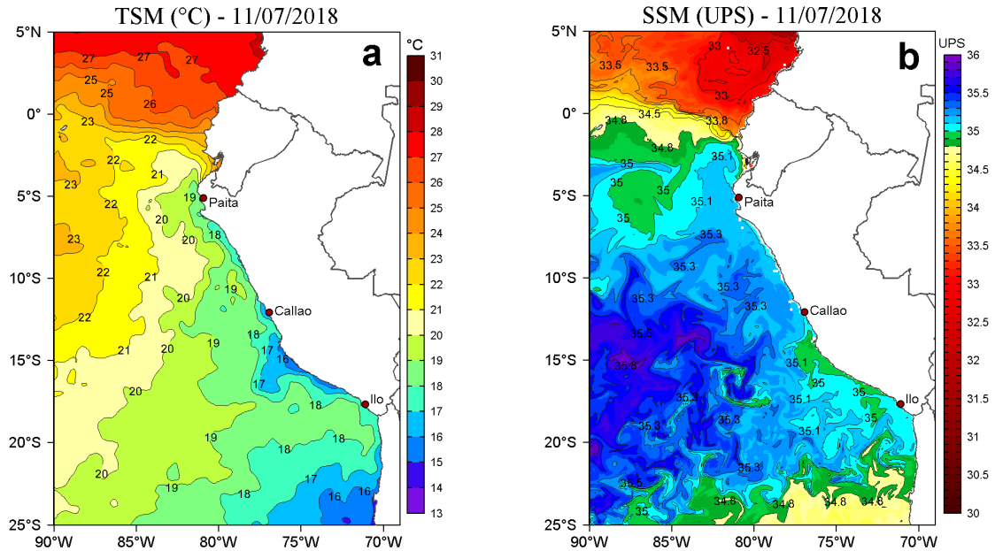
Figura 2. a) Temperatura Superficial del Mar ( ^{\circ}\text{C} ) y b) Salinidad Superficial del Mar (UPS) para el 11 de julio de 2018. Datos: OSTIA-UKMO-L4-GLOB-v2.0 (UK Met Office, 2012; Donlon et al, 2012) disponible en https://podaac.jpl.nasa.gov/dataset/OSTIA-UKMO-L4-GLOB-v2.0 para (a) y Hybrid Coordinate Ocean Model (HYCOM; Halliwell et al., 1998; 2000; Bleck, 2001) para (b). Procesamiento: LHFM/AFIOF/DGIOCC/IMARPE.
