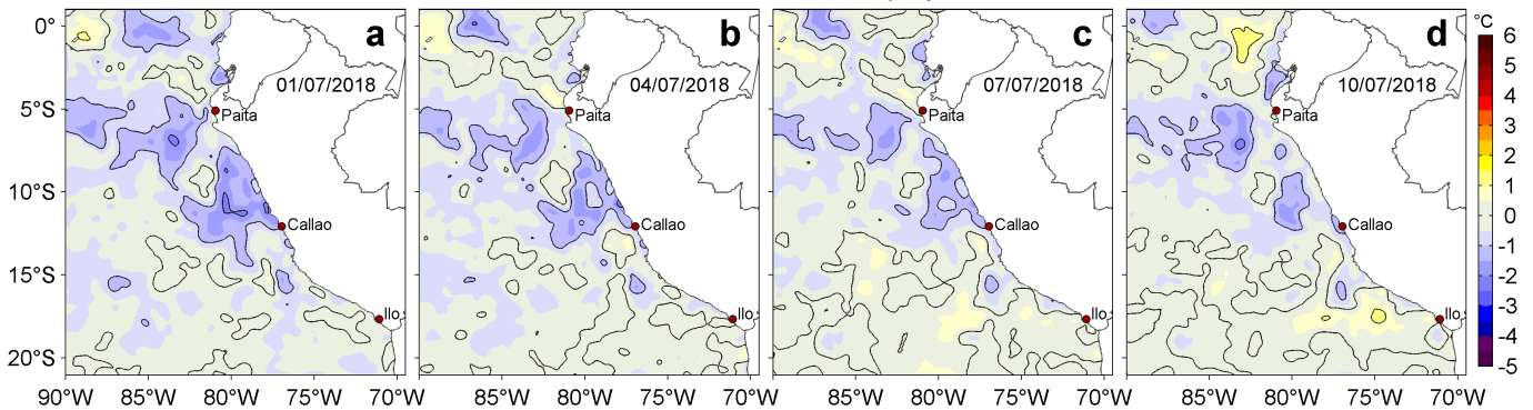
Figura 3. Anomalías de la Temperatura Superficial del Mar ( ^{\circ}\text{C} ) para los días: a) 01, b) 04, c) 07 y d) 10 de julio de 2018. Las anomalías se calcularon respecto de la climatología para el periodo 2007-2016. Datos: OSTIA-UKMO-L4-GLOB-v2.0 (UK Met Office, 2012; Donlon et al, 2012). Procesamiento: LHF/AFIOF/DGIOCC/IMARPE.
