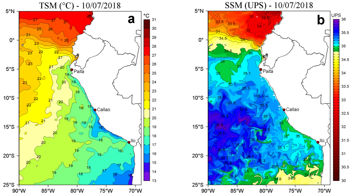
Figura 2. a) Temperatura Superficial del Mar ( ^{\circ}\text{C} ) y b) Salinidad Superficial del Mar (UPS) para el 10 de julio de 2018. Datos: OSTIA-UKMO-L4-GLOB-v2.0 (UK Met Office, 2012; Donlon et al, 2012) disponible en https://podaac.jpl.nasa.gov/dataset/OSTIA-UKMO-L4-GLOB-v2.0 para (a) y Hybrid Coordinate Ocean Model (HYCOM; Halliwell et al., 1998; 2000; Bleck, 2001) para (b). Procesamiento: LHF/AFIOF/DGIOCC/IMARPE.
