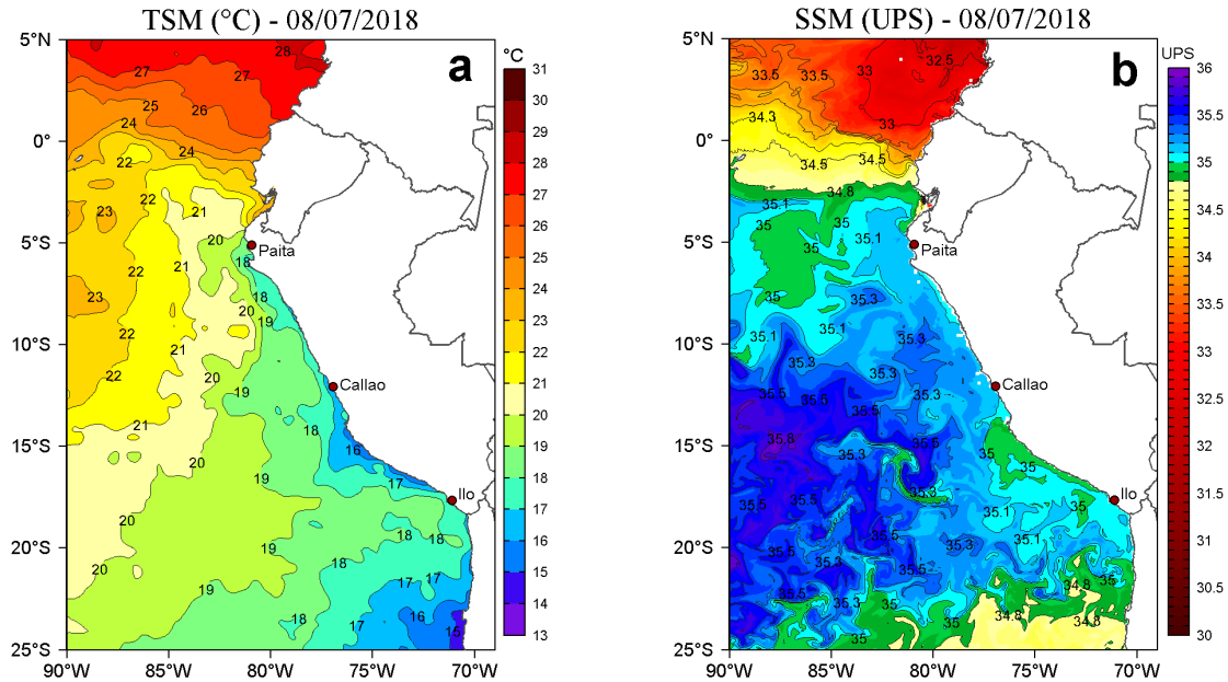
Figura 2. a) Temperatura Superficial del Mar (°C) y b) Salinidad Superficial del Mar (UPS) para el 08 de julio de 2018. Datos: OSTIA-UKMO-L4-GLOB-v2.0 (UK Met Office, 2012; Donlon et al, 2012) disponible en https://podaac.jpl.nasa.gov/dataset/OSTIA-UKMO-L4-GLOB-v2.0 para (a) y Hybrid Coordinate Ocean Model (HYCOM; Halliwell et al., 1998; 2000; Bleck, 2001) para (b). Procesamiento: LHF/AFIOF/DGIOCC/IMARPE.
