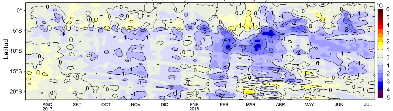
Figura 4. Variación promedio de las anomalías de la Temperatura Superficial del Mar (°C) para una franja de 60 mn (~111 km) adyacente al litoral peruano para los últimos doce meses al 08 de julio de 2018. Datos: OSTIA-UKMO-L4-GLOB-v2.0 (UK Met. Office, 2012; Donlon et al, 2012) disponible en https://podaac.jpl.nasa.gov/dataset/OSTIA-UKMO-L4-GLOB-v2.0 . Las anomalías se calcularon con respecto al periodo 2007-2016. Procesamiento: LHF/AFIOF/DGIOCC/IMARPE.
