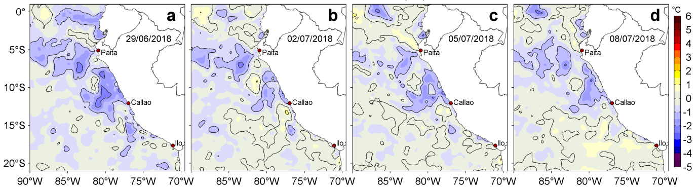
Figura 3. Anomalías de la Temperatura Superficial del Mar (°C) para los días: a) 29 de junio, b) 02, c) 05 y d) 08 de julio de 2018. Las anomalías se calcularon respecto de la climatología para el periodo 2007-2016. Datos: OSTIA-UKMO-L4-GLOB-v2.0 (UK Met Office, 2012; Donlon et al, 2012). Procesamiento: LHF/AFIOF/DGIOCC/IMARPE.
