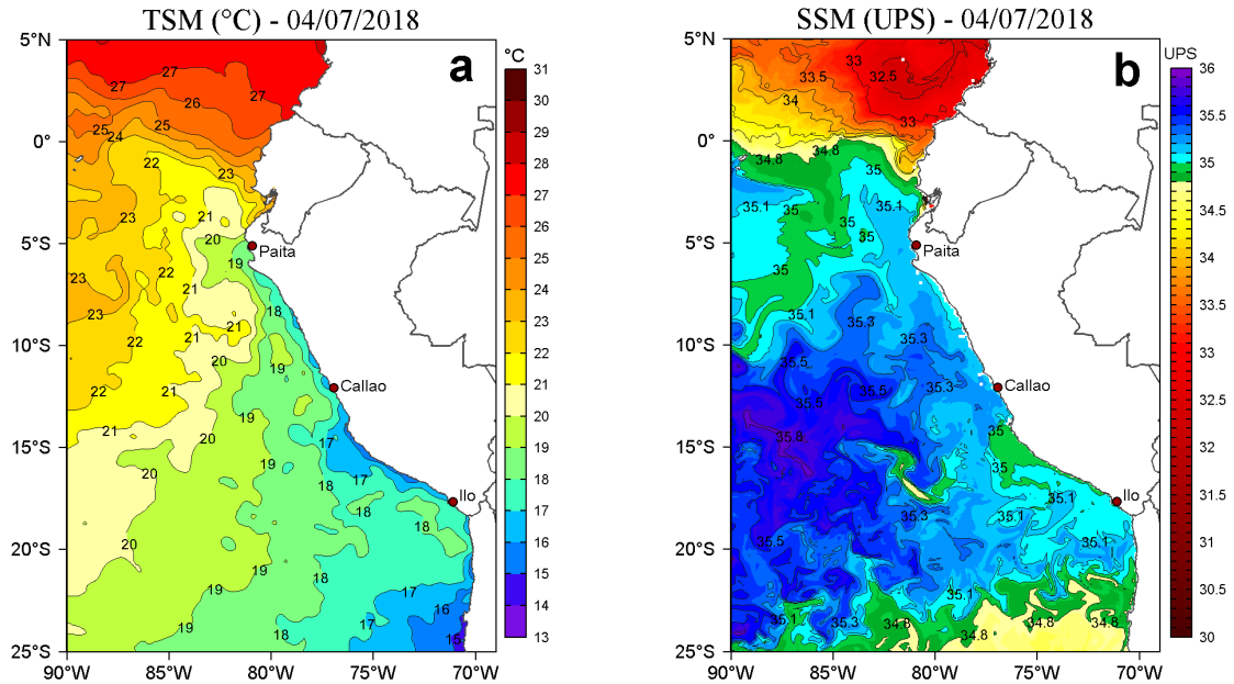
Figura 2. a) Temperatura Superficial del Mar ( ^{\circ}\text{C} ) y b) Salinidad Superficial del Mar (UPS) para el 04 de julio de 2018. Datos: OSTIA-UKMO-L4-GLOB-v2.0 (UK Met Office, 2012; Donlon et al, 2012) disponible en https://podaac.jpl.nasa.gov/dataset/OSTIA-UKMO-L4-GLOB-v2.0 para (a) y Hybrid Coordinate Ocean Model (HYCOM; Halliwell et al., 1998; 2000; Bleck, 2001) para (b). Procesamiento: LHF/AFIOF/DGIOCC/IMARPE.
