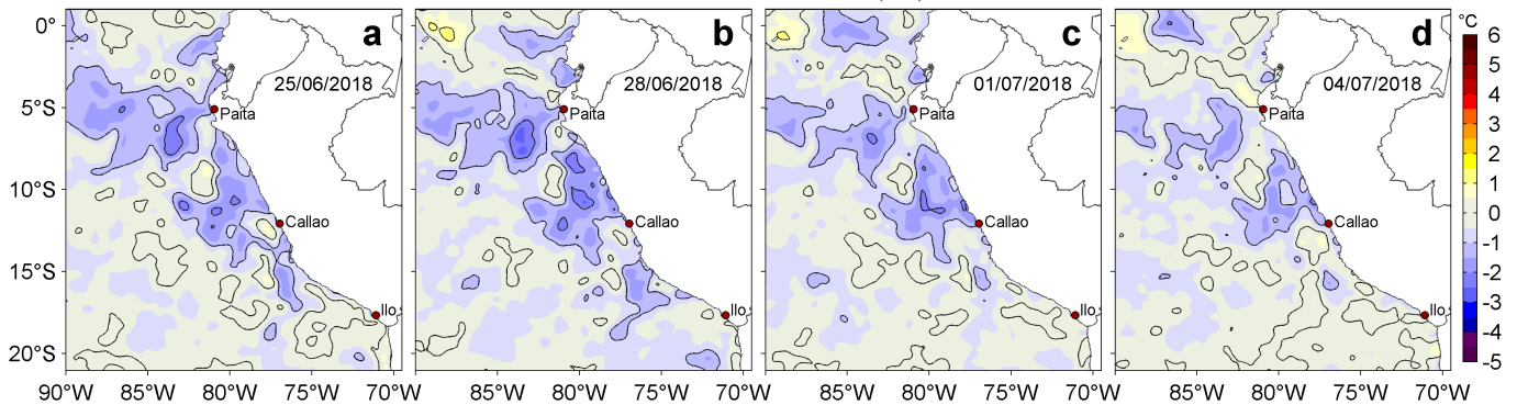
Figura 3. Anomalías de la Temperatura Superficial del Mar ( ^{\circ}\text{C} ) para los días: a) 25 y b) 28 de junio, c) 01 y d) 04 de julio de 2018. Las anomalías se calcularon respecto de la climatología para el periodo 2007-2016. Datos: OSTIA-UKMO-L4-GLOB-v2.0 (UK Met Office, 2012; Donlon et al, 2012). Procesamiento: LHF/AFIOF/DGIOCC/IMARPE.
