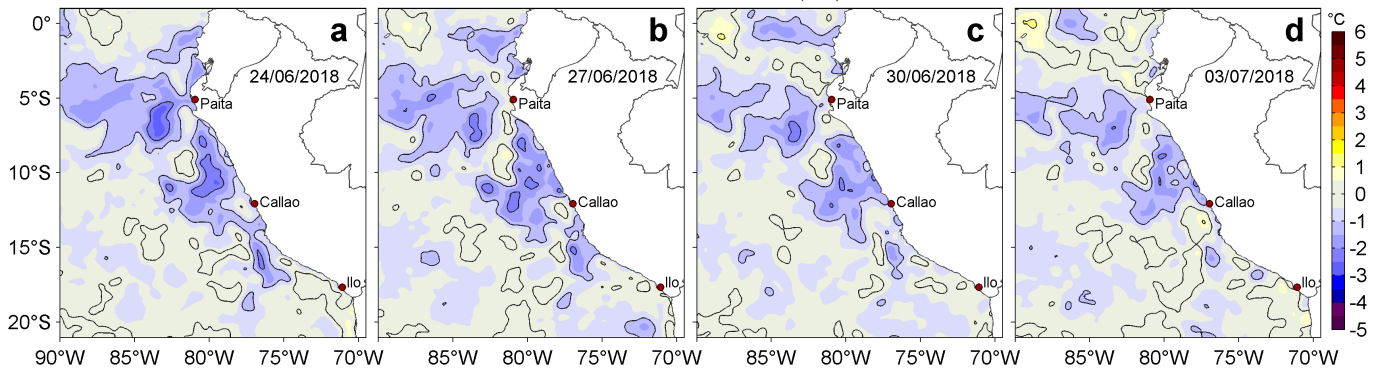
Figura 3. Anomalías de la Temperatura Superficial del Mar ( ^{\circ}\text{C} ) para los días: a) 24, b) 27 y c) 30 de junio y d) 03 de julio de 2018. Las anomalías se calcularon respecto de la climatología para el periodo 2007-2016. Datos: OSTIA-UKMO-L4-GLOB-v2.0 (UK Met Office, 2012; Donlon et al, 2012). Procesamiento: LHF/AFIOF/DGIOCC/IMARPE.
