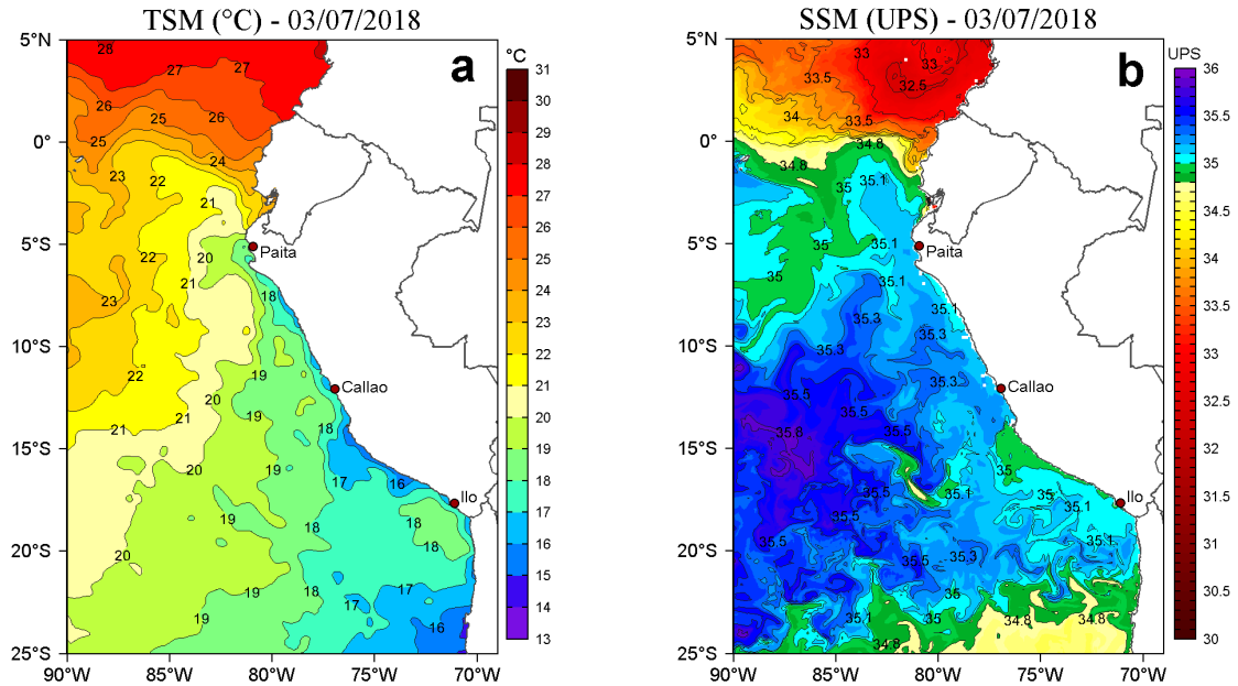
Figura 2. a) Temperatura Superficial del Mar ( ^{\circ}\text{C} ) y b) Salinidad Superficial del Mar (UPS) para el 03 de julio de 2018. Datos: OSTIA-UKMO-L4-GLOB-v2.0 (UK Met Office, 2012; Donlon et al, 2012) disponible en https://podaac.jpl.nasa.gov/dataset/OSTIA-UKMO-L4-GLOB-v2.0 para (a) y Hybrid Coordinate Ocean Model (HYCOM; Halliwell et al., 1998; 2000; Bleck, 2001) para (b). Procesamiento: LHF/AFIOF/DGIOCC/IMARPE.
