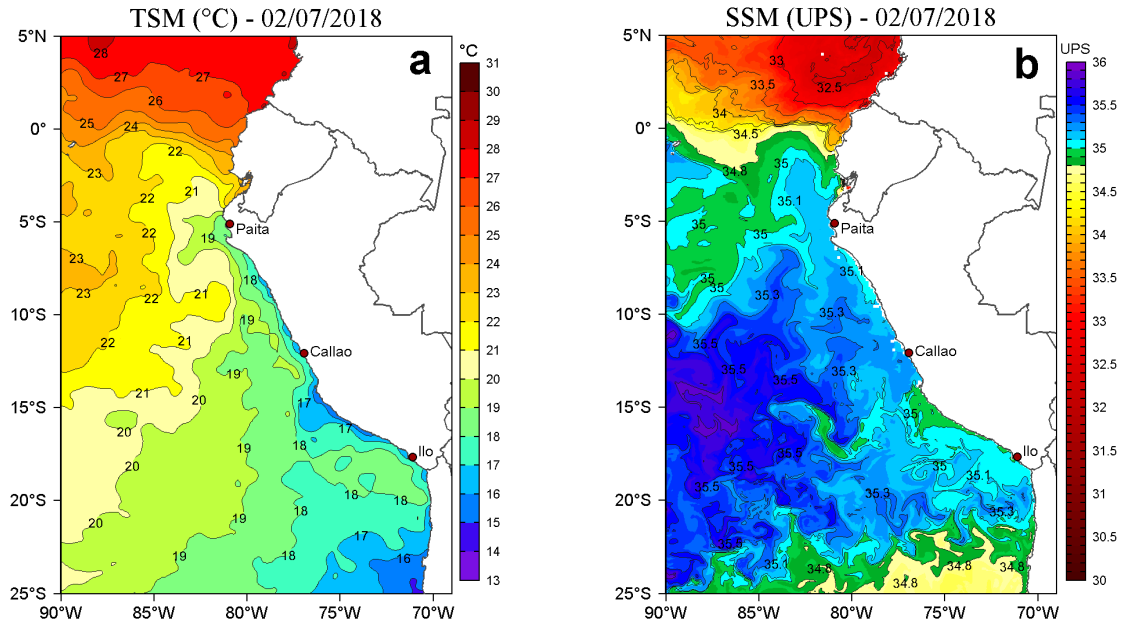
Figura 2. a) Temperatura Superficial del Mar ( ^{\circ}\text{C} ) y b) Salinidad Superficial del Mar (UPS) para el 02 de julio de 2018. Datos: OSTIA-UKMO-L4-GLOB-v2.0 (UK Met Office, 2012; Donlon et al, 2012) disponible en https://podaac.jpl.nasa.gov/dataset/OSTIA-UKMO-L4-GLOB-v2.0 para (a) y Hybrid Coordinate Ocean Model (HYCOM; Halliwell et al., 1998; 2000; Bleck, 2001) para (b). Procesamiento: LHF/AFIOF/DGIOCC/IMARPE.
