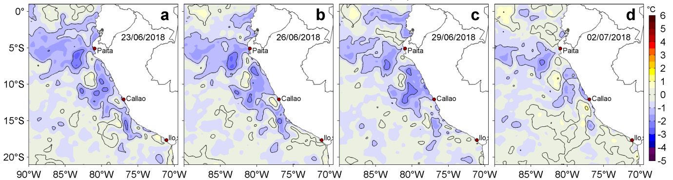
Figura 3. Anomalías de la Temperatura Superficial del Mar ( ^{\circ}\text{C} ) para los días: a) 23, b) 26 y c) 29 de junio y d) 02 de julio de 2018. Las anomalías se calcularon respecto de la climatología para el periodo 2007-2016. Datos: OSTIA-UKMO-L4-GLOB-v2.0 (UK Met Office, 2012; Donlon et al, 2012). Procesamiento: LHF/AFIOF/DGIOCC/IMARPE.
