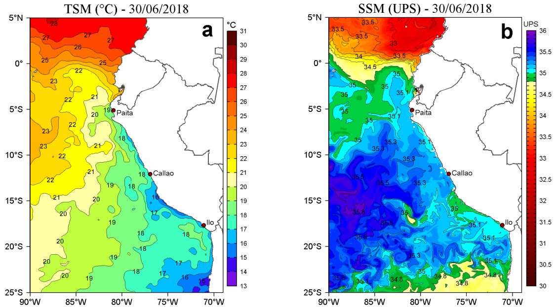
Figura 2. a) Temperatura Superficial del Mar ( ^{\circ}\text{C} ) y b) Salinidad Superficial del Mar (UPS) para el 30 de junio de 2018. Datos: OSTIA-UKMO-L4-GLOB-v2.0 (UK Met Office, 2012; Donlon et al, 2012) disponible en https://podaac.jpl.nasa.gov/dataset/OSTIA-UKMO-L4-GLOB-v2.0 para (a) y Hybrid Coordinate Ocean Model (HYCOM; Halliwell et al., 1998; 2000; Bleck, 2001) para (b). Procesamiento: LHF/AFIOF/DGIOCC/IMARPE.
