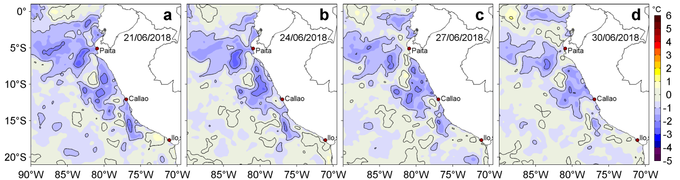
Figura 3. Anomalías de la Temperatura Superficial del Mar ( ^{\circ}\text{C} ) para los días: a) 21, b) 24, c) 27 y d) 30 de junio de 2018. Las anomalías se calcularon respecto de la climatología para el periodo 2007-2016. Datos: OSTIA-UKMO-L4-GLOB-v2.0 (UK Met Office, 2012; Donlon et al, 2012). Procesamiento: LHF/AFIOF/DGIOCC/IMARPE.
