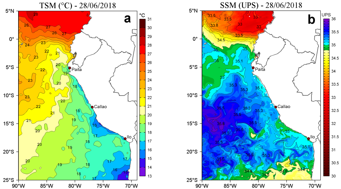
Figura 2. a) Temperatura Superficial del Mar ( ^{\circ}\text{C} ) y b) Salinidad Superficial del Mar (UPS) para el 28 de junio de 2018. Datos: OSTIA-UKMO-L4-GLOB-v2.0 (UK Met Office, 2012; Donlon et al, 2012) disponible en https://podaac.jpl.nasa.gov/dataset/OSTIA-UKMO-L4-GLOB-v2.0 para (a) y Hybrid Coordinate Ocean Model (HYCOM; Halliwell et al., 1998; 2000; Bleck, 2001) para (b). Procesamiento: LHF/AFIOF/DGIOCC/IMARPE.
