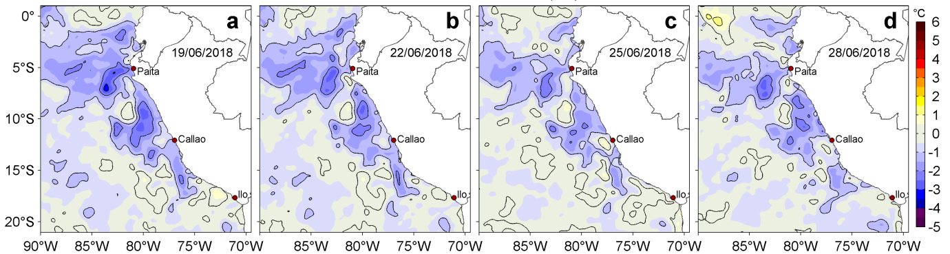
Figura 3. Anomalías de la Temperatura Superficial del Mar ( ^{\circ}\text{C} ) para los días: a) 19, b) 22, c) 25 y d) 28 de junio de 2018. Las anomalías se calcularon respecto de la climatología para el periodo 2007-2016. Datos: OSTIA-UKMO-L4-GLOB-v2.0 (UK Met Office, 2012; Donlon et al, 2012). Procesamiento: LHF/AFIOF/DGIOCC/IMARPE.
