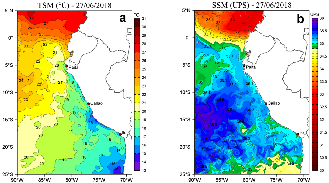
Figura 2. a) Temperatura Superficial del Mar ( ^{\circ}\text{C} ) y b) Salinidad Superficial del Mar (UPS) para el 27 de junio de 2018. Datos: OSTIA-UKMO-L4-GLOB-v2.0 (UK Met Office, 2012; Donlon et al, 2012) disponible en https://podaac.jpl.nasa.gov/dataset/OSTIA-UKMO-L4-GLOB-v2.0 para (a) y Hybrid Coordinate Ocean Model (HYCOM; Halliwell et al., 1998; 2000; Bleck, 2001) para (b). Procesamiento: LHF/AFIOF/DGIOCC/IMARPE.
