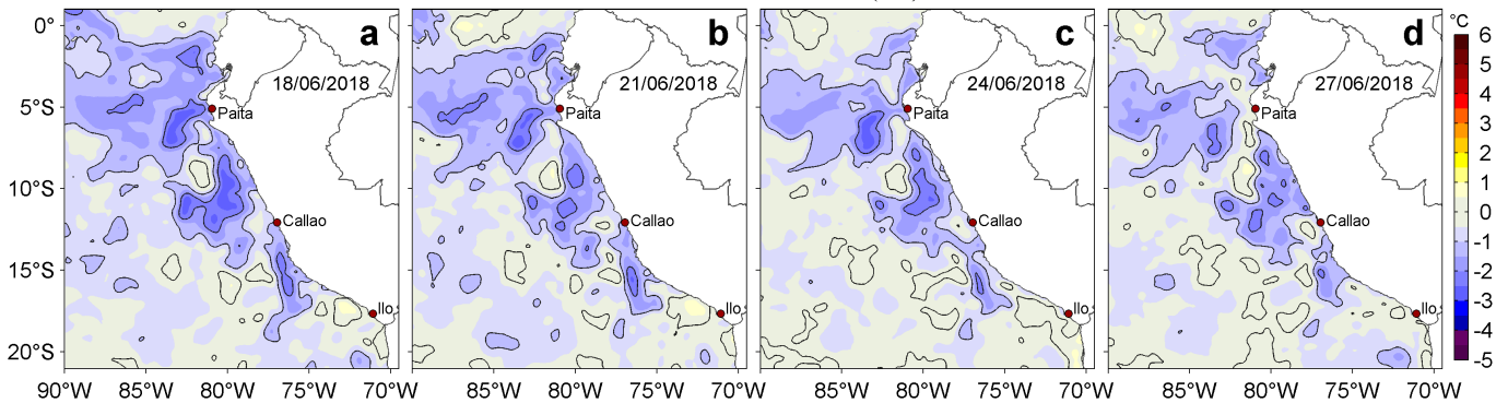
Figura 3. Anomalías de la Temperatura Superficial del Mar ( ^{\circ}\text{C} ) para los días: a) 18, b) 21, c) 24 y d) 27 de junio de 2018. Las anomalías se calcularon respecto de la climatología para el periodo 2007-2016. Datos: OSTIA-UKMO-L4-GLOB-v2.0 (UK Met Office, 2012; Donlon et al, 2012). Procesamiento: LHF/AFIOF/DGIOCC/IMARPE.
