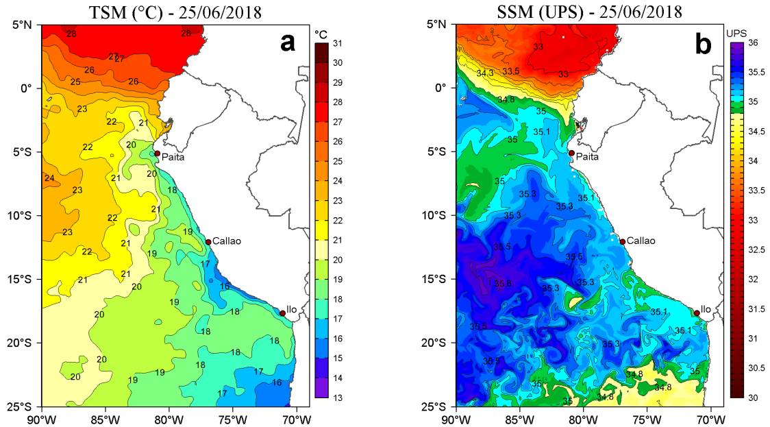
Figura 2. a) Temperatura Superficial del Mar ( ^{\circ}\text{C} ) y b) Salinidad Superficial del Mar (UPS) para el 25 de junio de 2018. Datos: OSTIA-UKMO-L4-GLOB-v2.0 (UK Met Office, 2012; Donlon et al, 2012) disponible en https://podaac.jpl.nasa.gov/dataset/OSTIA-UKMO-L4-GLOB-v2.0 para (a) y Hybrid Coordinate Ocean Model (HYCOM; Halliwell et al., 1998; 2000; Bleck, 2001) para (b). Procesamiento: LHF/AFIOF/DGIOCC/IMARPE.
