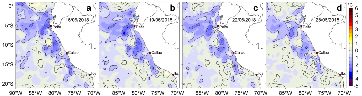
Figura 3. Anomalías de la Temperatura Superficial del Mar ( ^{\circ}\text{C} ) para los días: a) 16, b) 19, c) 22 y d) 25 de junio de 2018. Las anomalías se calcularon respecto de la climatología para el periodo 2007-2016. Datos: OSTIA-UKMO-L4-GLOB-v2.0 (UK Met Office, 2012; Donlon et al, 2012). Procesamiento: LHF/AFIOF/DGIOCC/IMARPE.
