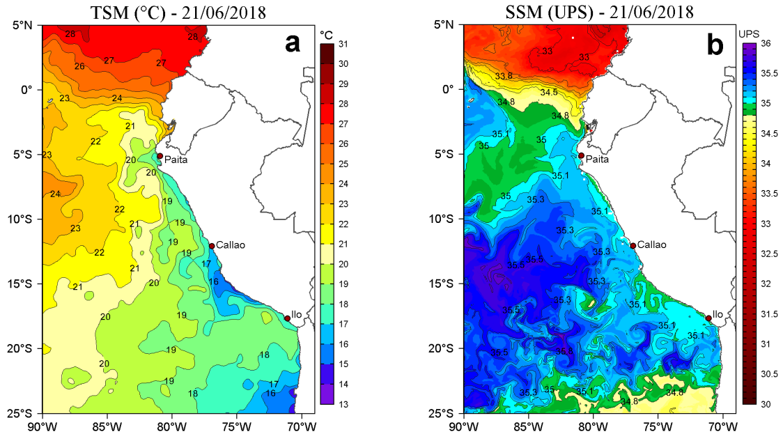
Figura 2. a) Temperatura Superficial del Mar (°C) y b) Salinidad Superficial del Mar (UPS) para el 21 de junio de 2018. Datos: OSTIA-UKMO-L4-GLOB-v2.0 (UK Met Office, 2012; Donlon et al, 2012) disponible en https://podaac.jpl.nasa.gov/dataset/OSTIA-UKMO-L4-GLOB-v2.0 para (a) y Hybrid Coordinate Ocean Model (HYCOM; Halliwell et al., 1998; 2000; Bleck, 2001) para (b). Procesamiento: LHF/AFIOF/DGIOCC/IMARPE.
