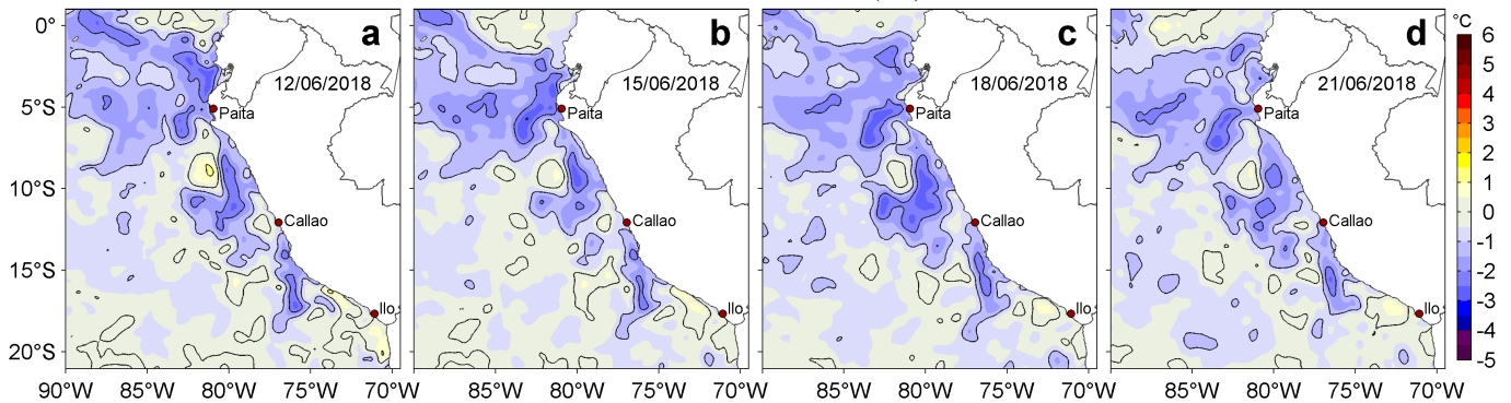
Figura 3. Anomalías de la Temperatura Superficial del Mar (°C) para los días: a) 12, b) 15, c) 18 y d) 21 de junio de 2018. Las anomalías se calcularon respecto de la climatología para el periodo 2007-2016. Datos: OSTIA-UKMO-L4-GLOB-v2.0 (UK Met Office, 2012; Donlon et al, 2012). Procesamiento: LHF/AFIOF/DGIOCC/IMARPE.
