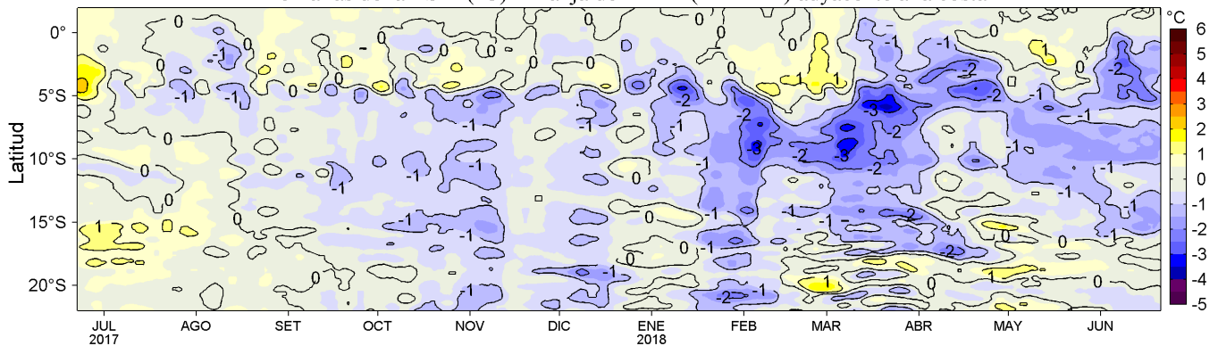
Figura 4. Variación promedio de las anomalías de la Temperatura Superficial del Mar (°C) para una franja de 60 mn (~111 km) adyacente al litoral peruano para los últimos doce meses al 21 de junio de 2018. Datos: OSTIA-UKMO-L4-GLOB-v2.0 (UK Met. Office, 2012; Donlon et al, 2012) disponible en https://podaac.jpl.nasa.gov/dataset/OSTIA-UKMO-L4-GLOB-v2.0 . Las anomalías se calcularon con respecto al periodo 2007-2016. Procesamiento: LHF/AFIOF/DGIOCC/IMARPE.
